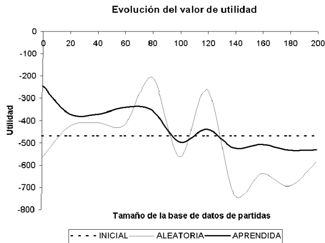
Figura 7. Evolución del valor de utilidad conforme aumenta el tamaño de la base de datos
