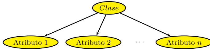
Figura 2. Topología de un clasificador Naive Bayes
