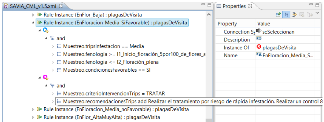
Fig. 1. Ejemplo de regla que evalúa el criterio de intervención para los trips
