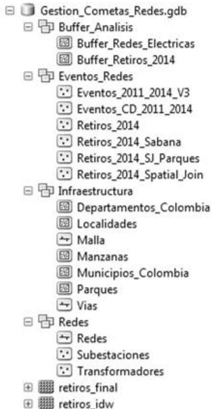
Figura 2. Gráfico GDB Gestion_Cometas_Red.es
