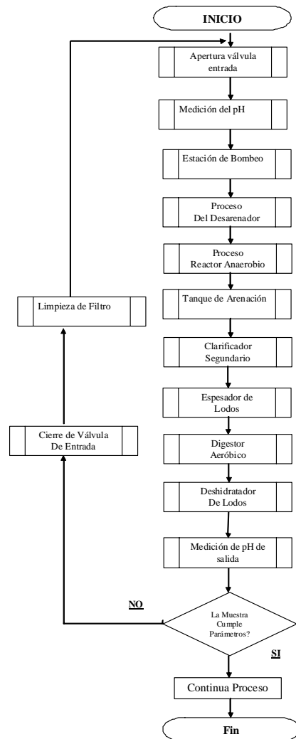
Fig. 6. Diagrama de Flujo PTAR. – Fuente: Elaborado por grupo de investigación. Junio de 2011
