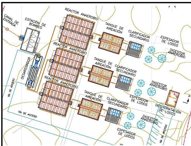
Fig. 7. Plano General de la Planta de Tratamiento de Aguas Residuales - PTAR. Fuente: Elaborado por grupo de investigación. Junio de 2011
