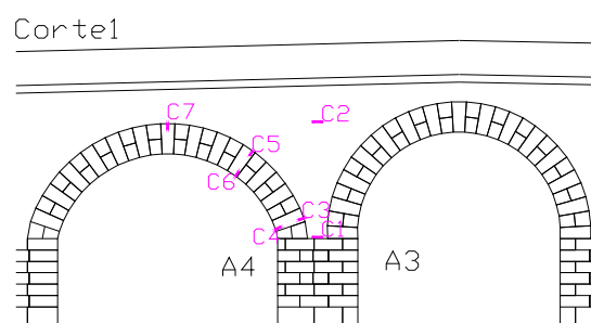
Fig 15- Posicionamento de células de pressão.
