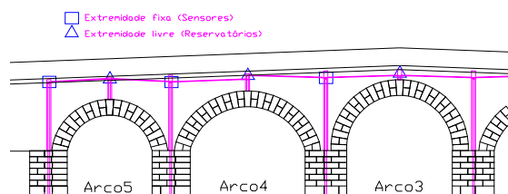
Fig 6a- Posicionamento dos sensores de pressão (corte longitudinal parcial de meia-ponte).
