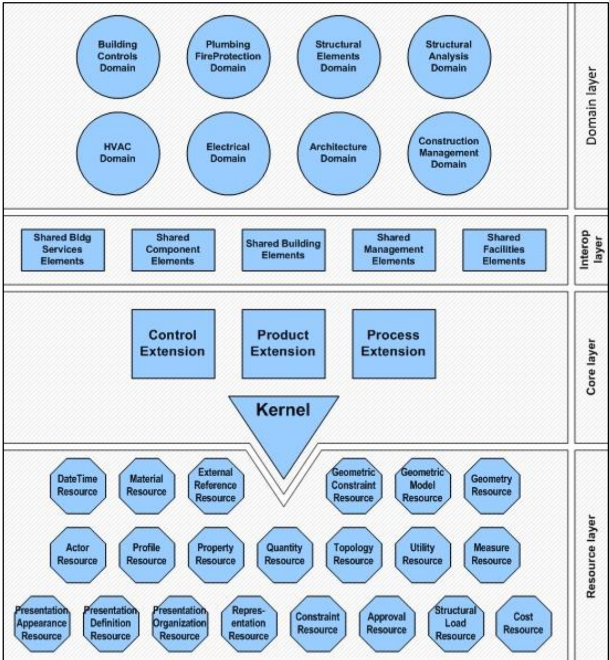
Figura 9 - Esquema da estrutura do IFC4 [Retirado de (buildingSMART, 2015)]
