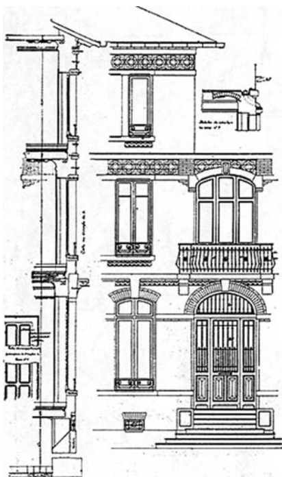
Casas geminadas H. dos Santos, detalhe construtivo, Ventura Terra, 1904
