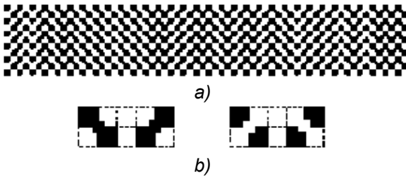
Figura 19 - Técnica de projecção de um padrão binário (imagens retiradas de [3]): a) Padrão binário usado por Vuylsteke e Oosterlinck ; b) Constituintes básicos desse padrão, ampliados.
