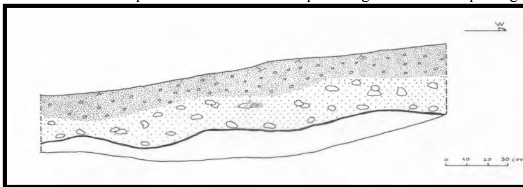
Perfil Sur Operación SB 20J-1 (Dibujo: C. Escobar Durand)
