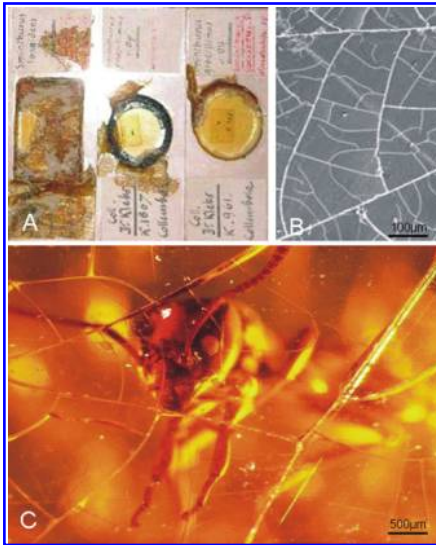
Abbildung 1: Versprödung von Bernsteinobjekten aus der Königsberger Bernsteinsammlung. A: Eingebettete Inklusionspräparate mit Verwitterungserscheinungen am Einbettungsmaterial (Kanadabalsam); B: Bernsteinoberfläche mit Craquelé-Struktur (FEM-Aufnahme); C: Bernstein mit Inkluse und oberflächlicher Rissbildung
