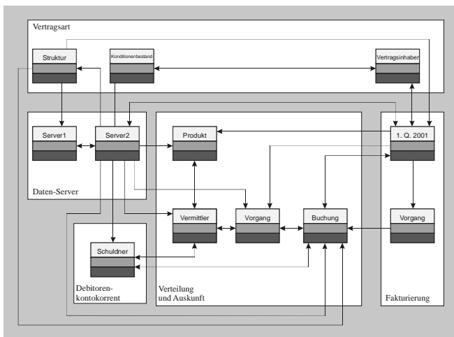
Abb. 9. Geschäftsprozessmodell
