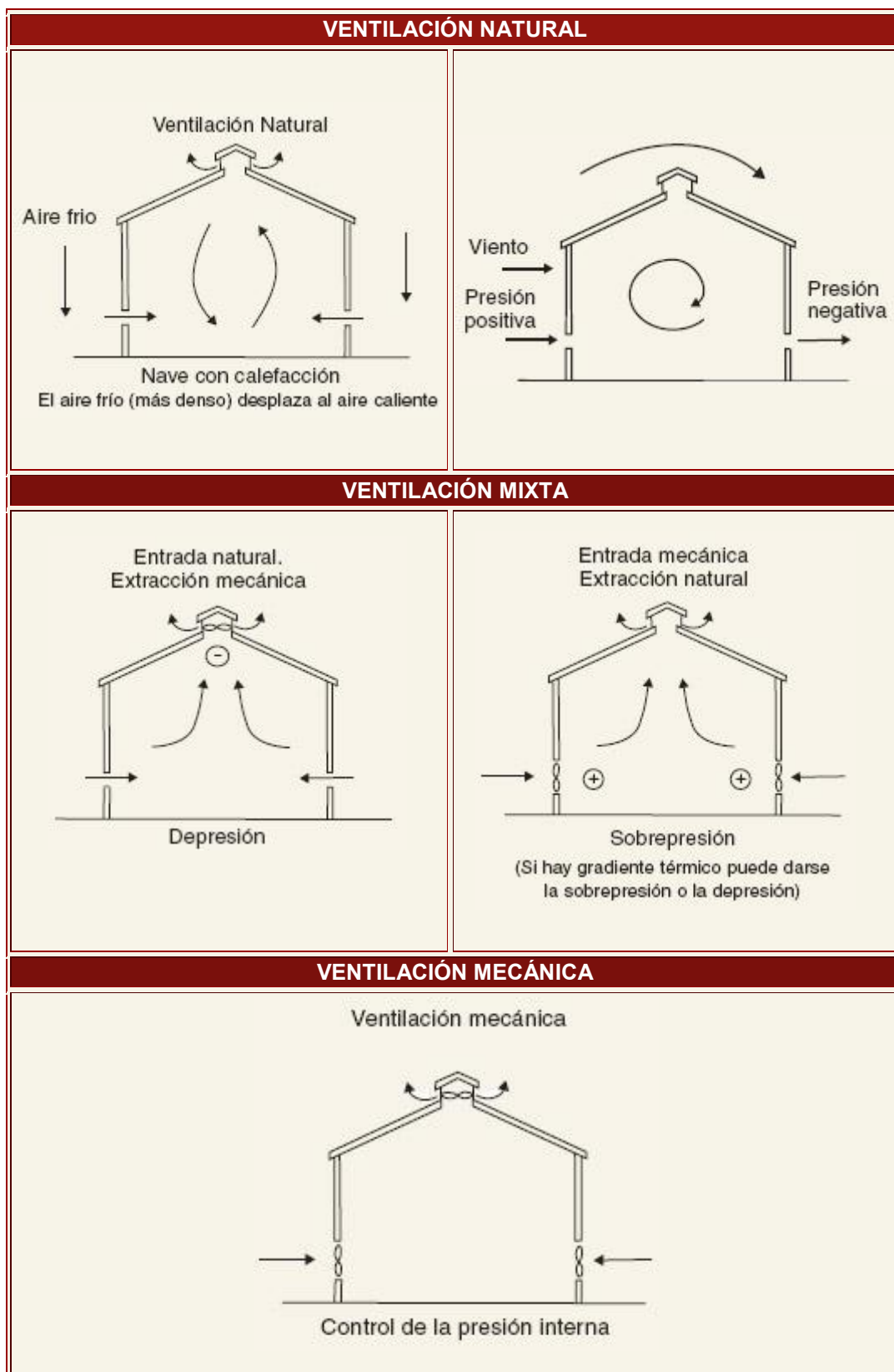
FIGURA 28. Ventilación natural vs. ventilación mecánica (Cavallé y Hernández, 2007).
