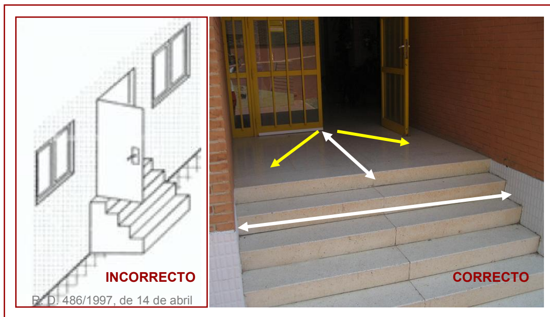
FIGURA 6. Puertas de acceso a una escalera con apertura hacia el exterior, sobre descanso adecuado, que forman parte de la vía de comunicación con las instalaciones deportivas de un centro público.
