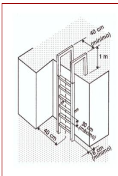
FIGURA 12. Esquema y dimensiones de una escala fija (R. D. 486/1997).
