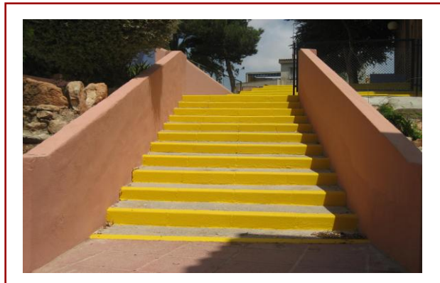
FIGURA 1. Escaleras señalizadas en vía de comunicación con las instalaciones deportivas de un centro público.
