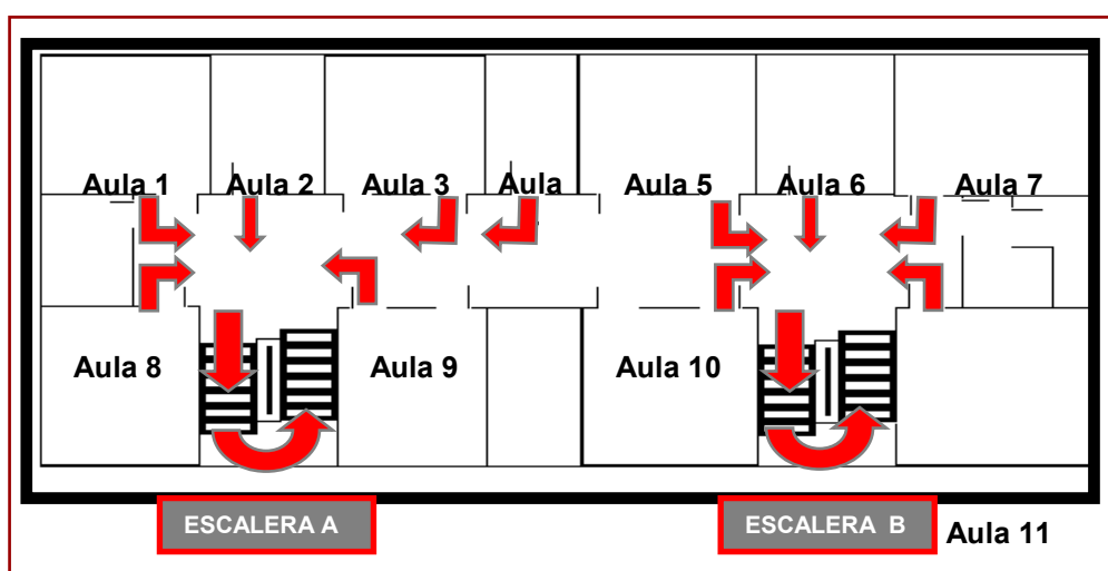
FIGURA 20. Esquema de flujos de evacuación de planta. Planta 1ª. Edificio 2. C.E.I.P. Fernando Garrido. Canteras – Cartagena (Rosique, 2009).
