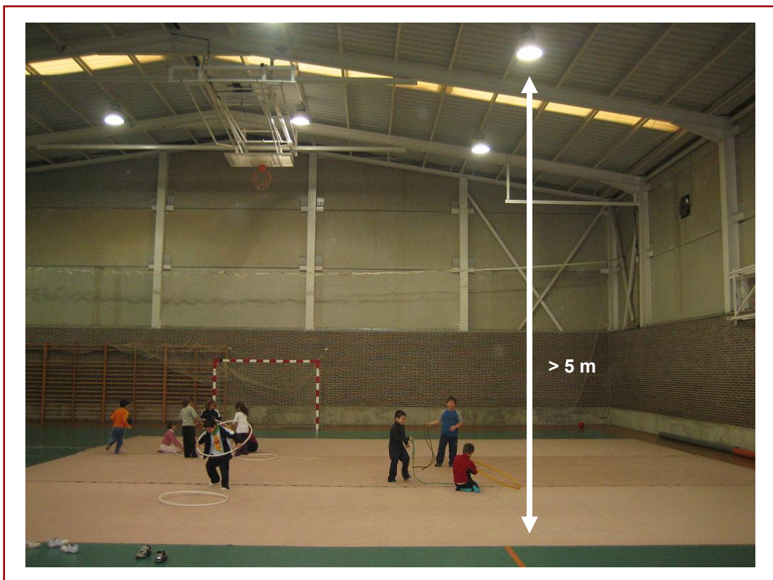
FIGURA 31. Ubicación de las luminarias en pabellón polideportivo municipal de uso escolar. Detalle de apantallamiento y altura de dichos elementos.
