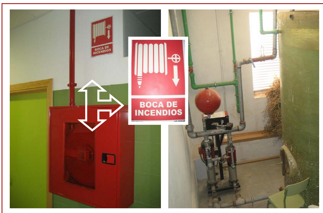
FIGURA 15. Bomba de presión, depósito auxiliar de agua y BIE (Boca de Incendios Equipada), adecuadamente señalizada, en centro público.
