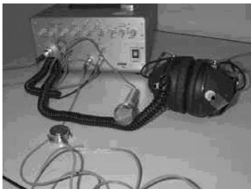
Figura 9. Suvag II con micrófono, auriculares y vibrador.
