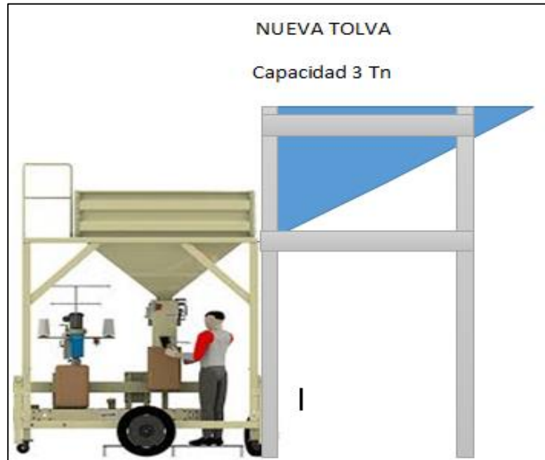
Figura 17 Nueva tolva de ensaque
