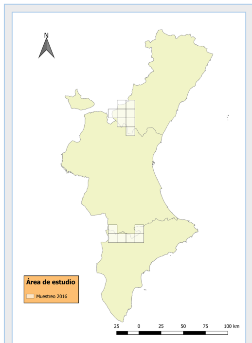
FIGURA 2. Área de estudio. Cuadrículas UTM 10x10 muestreadas en el presente trabajo.
