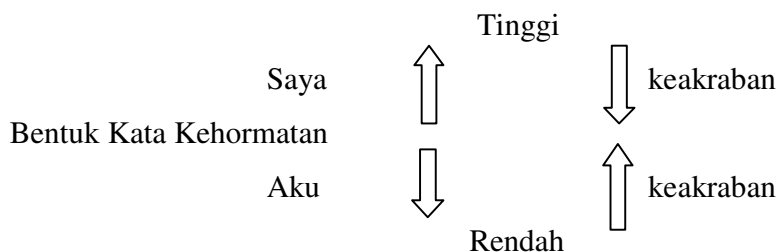
Rajah 2. Tahap kehormatan ganti nama 'saya' dan 'aku'
