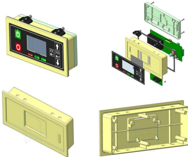
Рисунок – Компоновання корпусу контролера та зовнішній вигляд корпусних деталей
