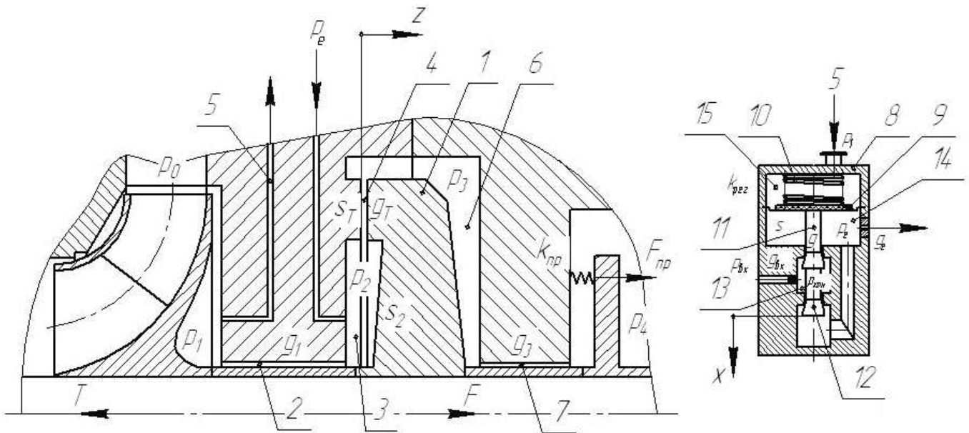
Рисунок 5 – Запірно-рівноважуючий пристрій:
