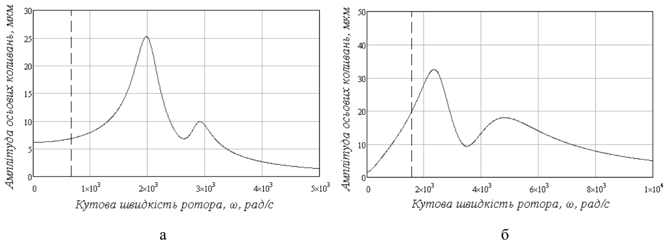
Рисунок 8 – Амплітудні частотні характеристики ротора насоса (а) і компресора (б)
