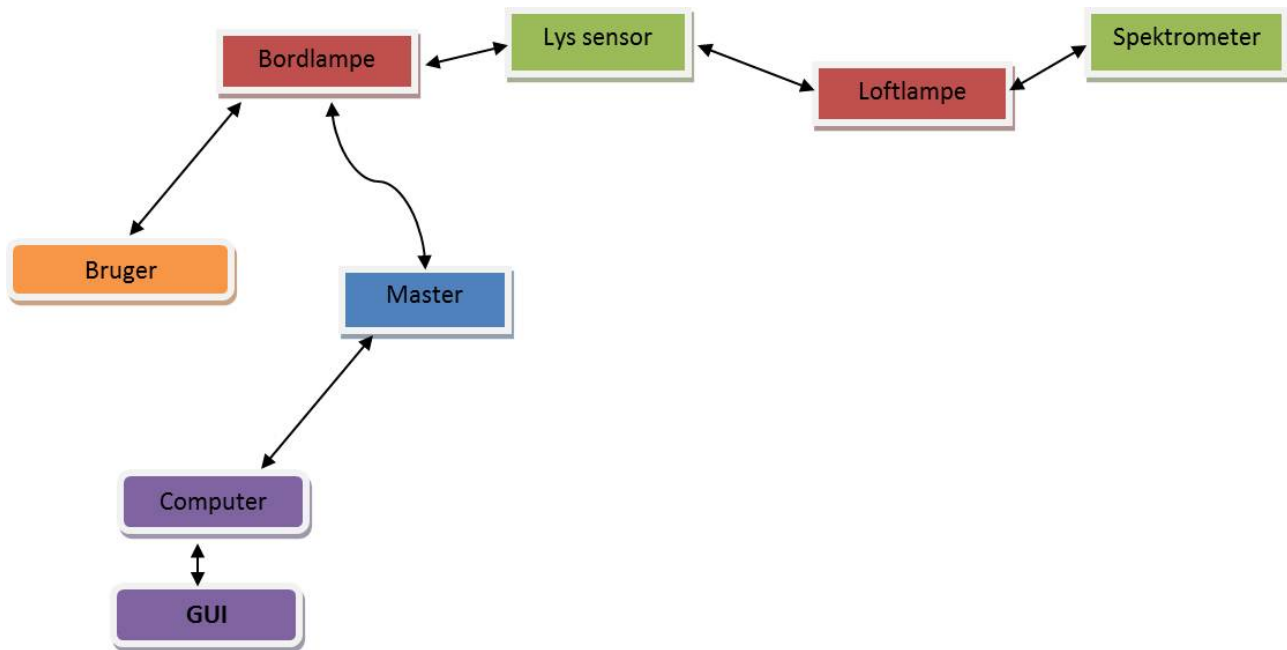
Figur 15 Skematisk tegning af det intelligente dynamiske belysningsystem.
