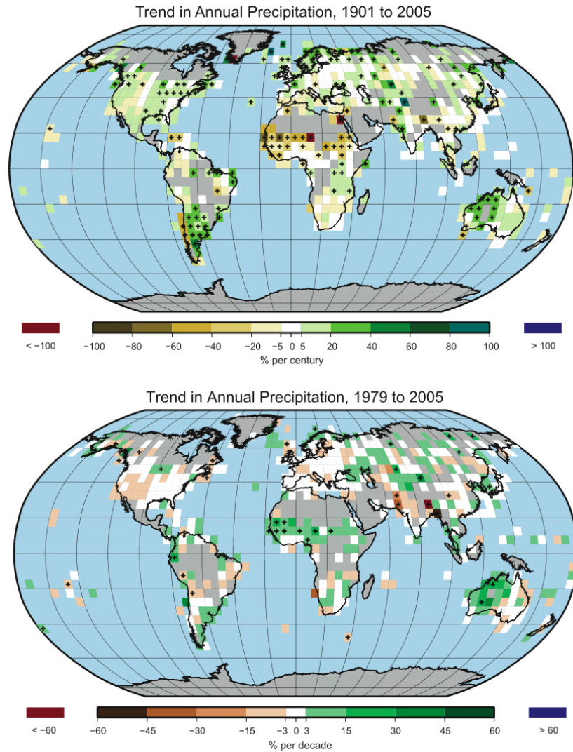
Figur 1. Tendenser i årlig nedbør i procent per århundrede for perioden 1901 til 2005 (øverst) og per årti for 1979 til 2005 (nederst), baseret på GHCN nedbørsdata fra NCDC. Procenterne er beregnet i forhold til perioden 1961 til 1990. Områder vist med grå farve har ikke data nok til at kunne beregne en pålidelig tendens. Kilde: (IPCC, 2007).
