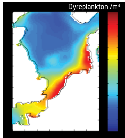
Figur 18. Årgennemsnit for biomasser af dyreplankton i Nordsøen. Figuren viser, at der er mest dyreplankton i den syd-østlige del af Nordsøen.
