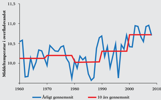
Figur 1. Middelttemperaturen i overfladevandet i Nordsøen fra 1960-2010 vist for hvert år (blå) og som gennemsnit over 10 år (rød).
