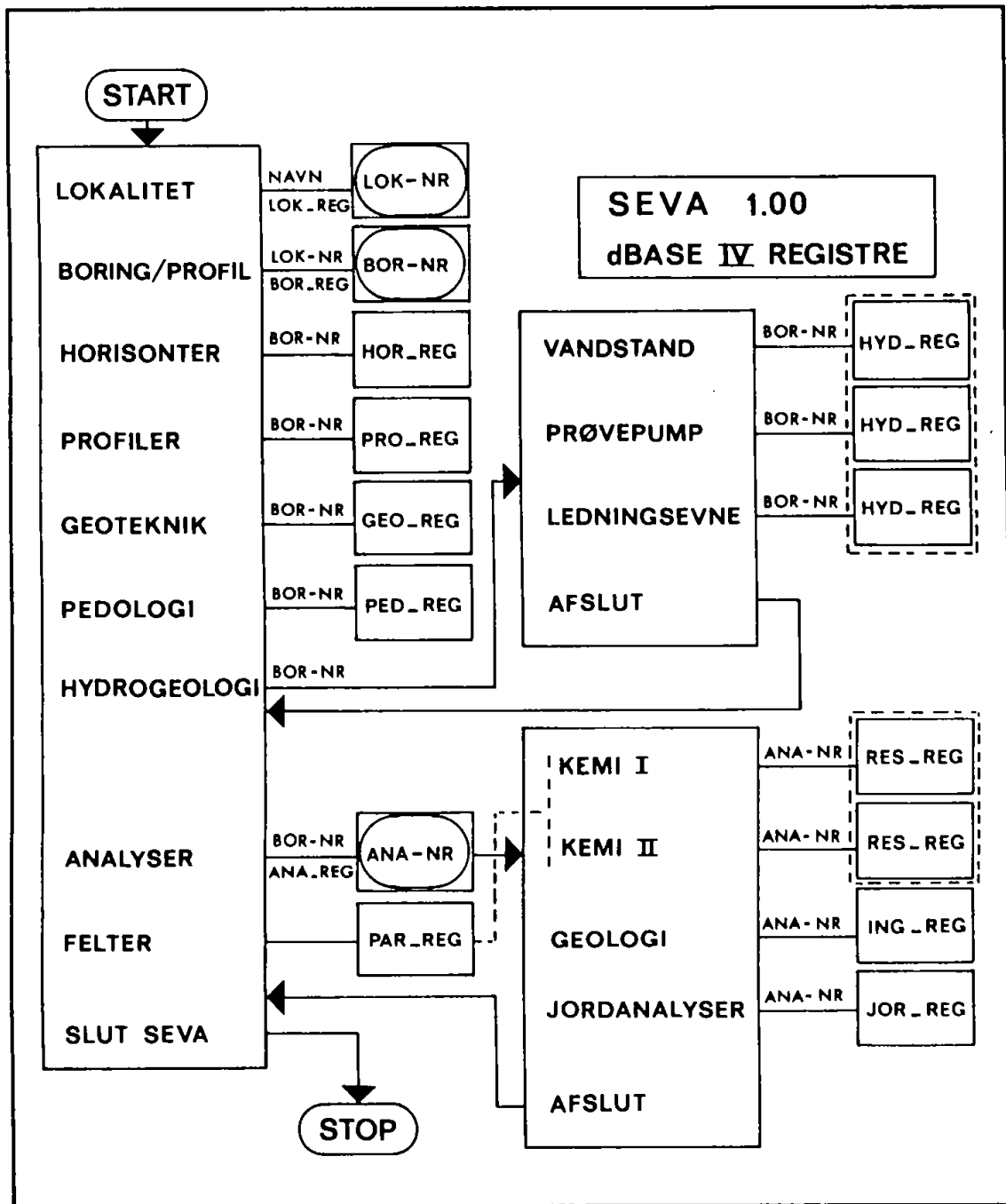
Figur 1: Datastruktur for SeVa
