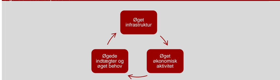
Figur 6.3 Kausalitetsproblemet
