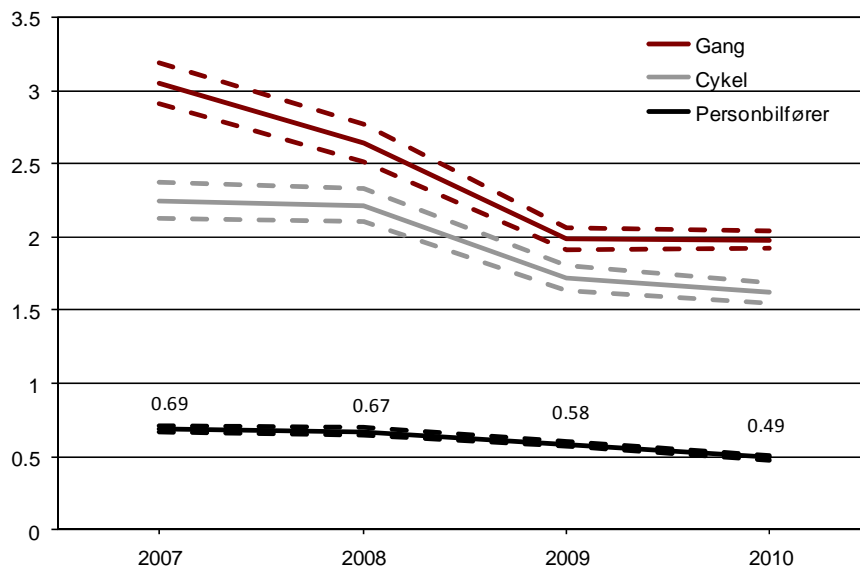
Figur 12 Totalrisiko 2007-2010 for gang, cykel og personbilfører (dræbte og alvorligt skadede per 10 mio. km)
