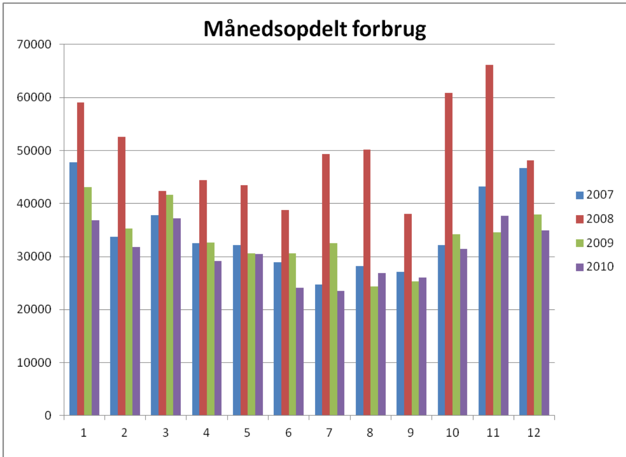
Figur 4 Månedsopdelt elforbrug for de seneste fire år (Opdateres når data foreligger)
