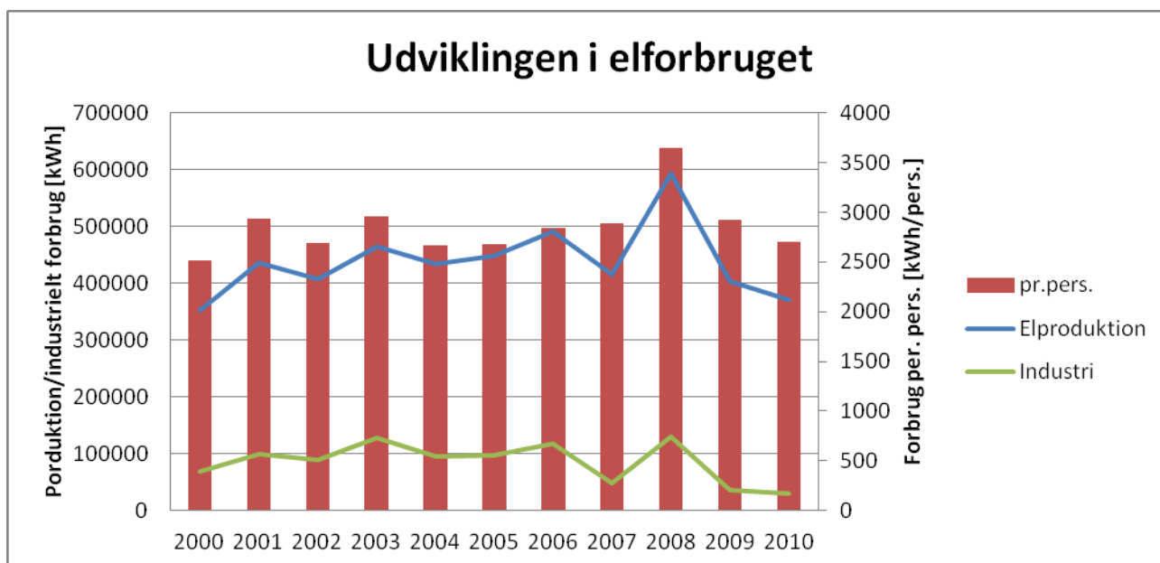
Figur 3 Elproduktionen i Sarfannguaq, det industrielle forbrug og forbruget per person exkl. industriel de sidste ti år
