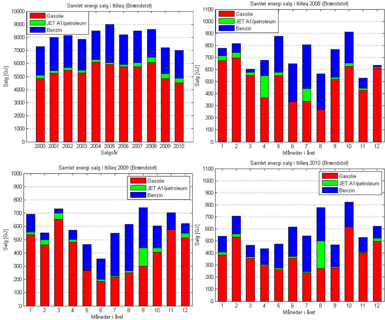
Figur 19 Brændstofsalg omregnet til energisalg
