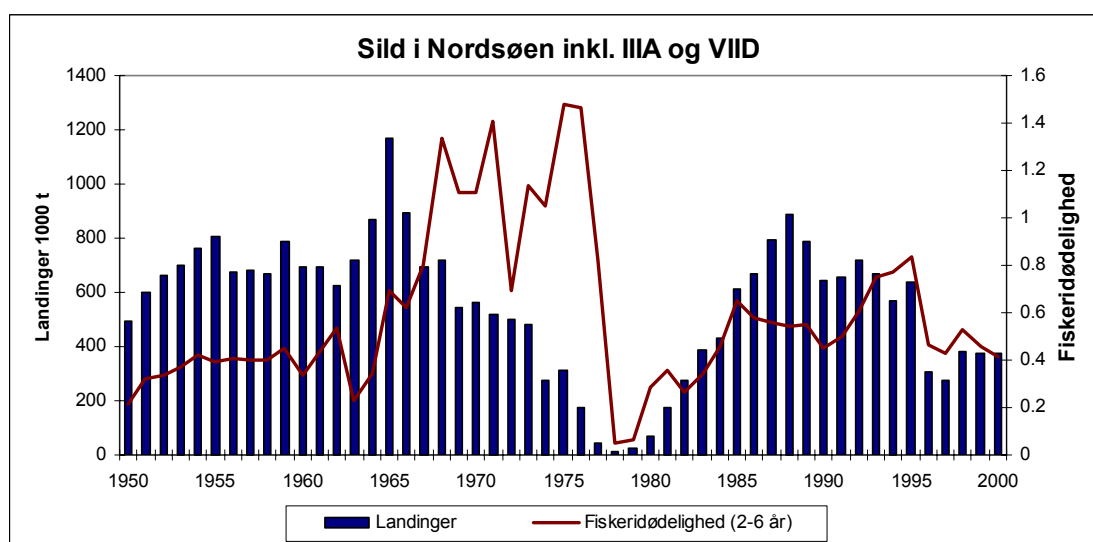
Fig. 2.1.1. Sild i Nordsøen: Landinger og fiskeridødelighed
