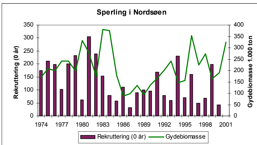
Figur 13.1.2. Sperling i Nordsøen og Skagerrak. Udvikling i rekruttering og gydebiomasse.
