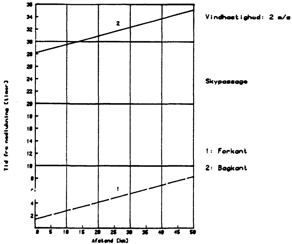
Fig. 4.2. Tidsforløb for skypassage med vindhastighed 2 m/s, som bruges ved stabilitet F.
