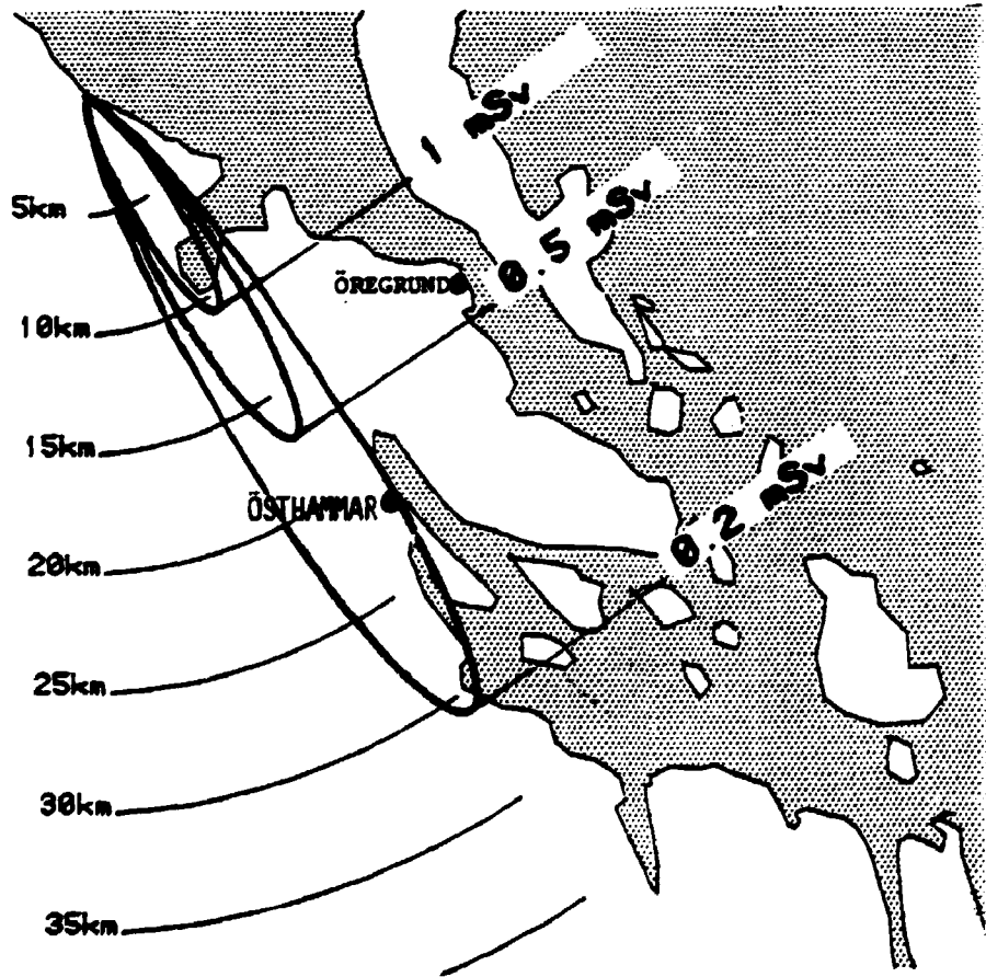
Fig. C.13. Gammadosis fra deponeret aktivitet efter 1 år. Efter det tørste 1 1/2 døgn indendørs regnes med normal færden i 365 dage på det pågældende sted.
