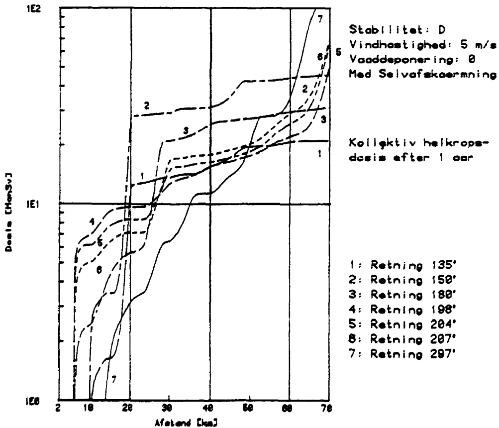
Fig. C.15. Kollektiv helkropsdosis som funktion af afstanden fra værket i de 7 udslipsretninger, hvor kollektivdosis er størst.
