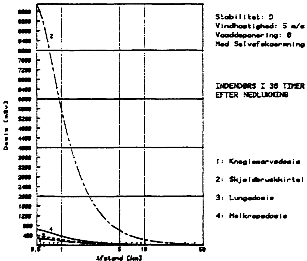
Fig. 5.3. Organdoser ved 36 timers indendørs ophold.
