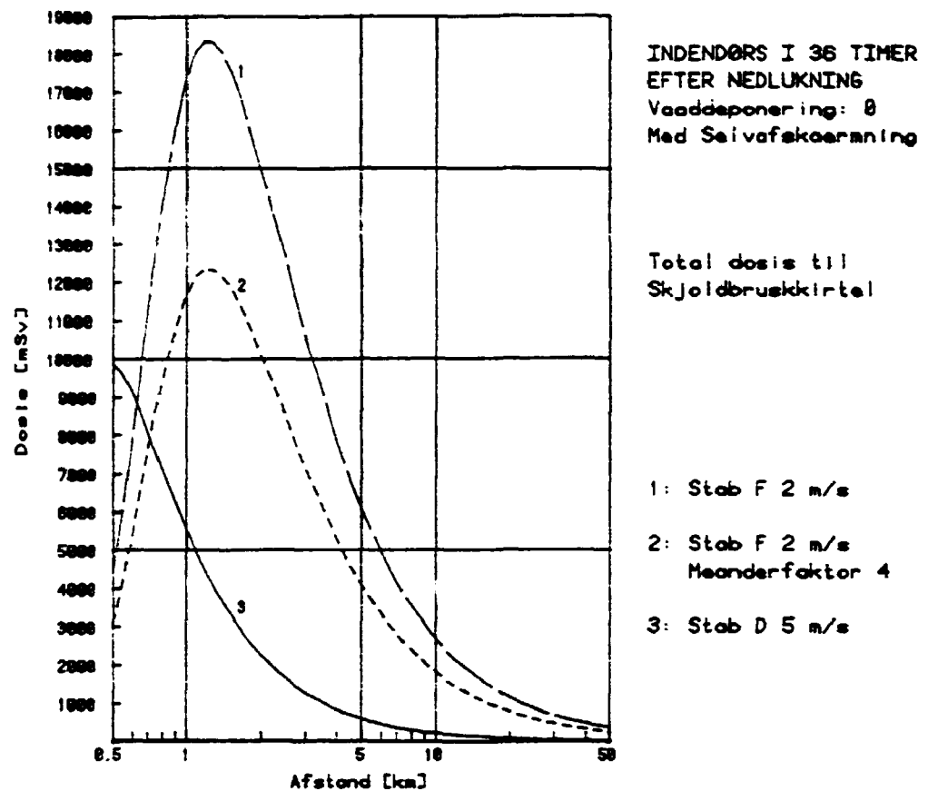
Fig. C.3. Total skjoldbruskkirteldosis ved stabilitet F og D.
