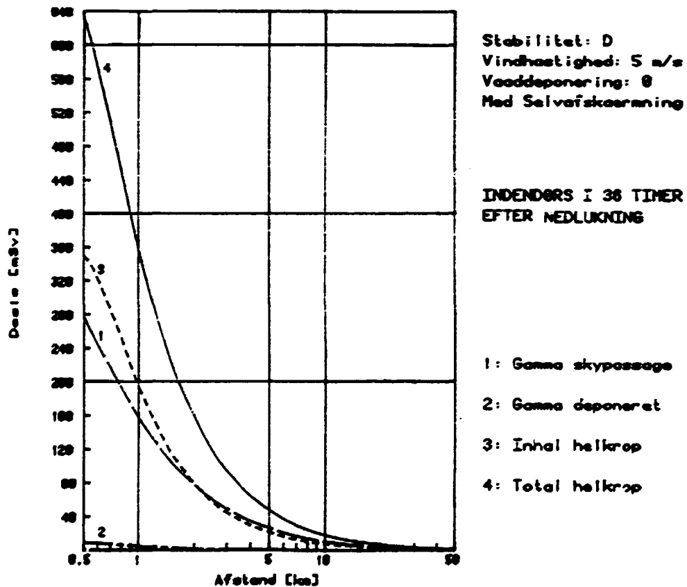
Fig. 5.1. Total helkropsdosis i skyens centerlinie opdelt i dosiskomponenter.
