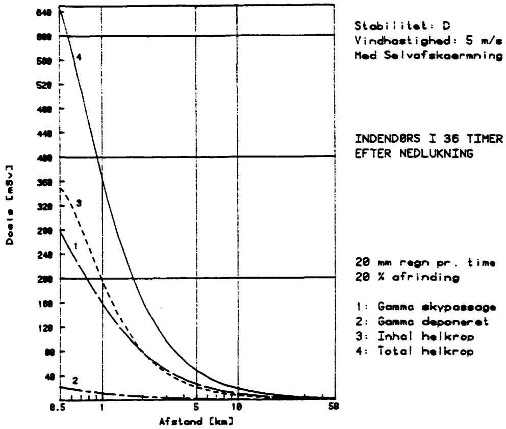
Fig. 5.6. Total helkropsdosis opdelt i dosiskomponenter ved 20 mm regn i timen.
