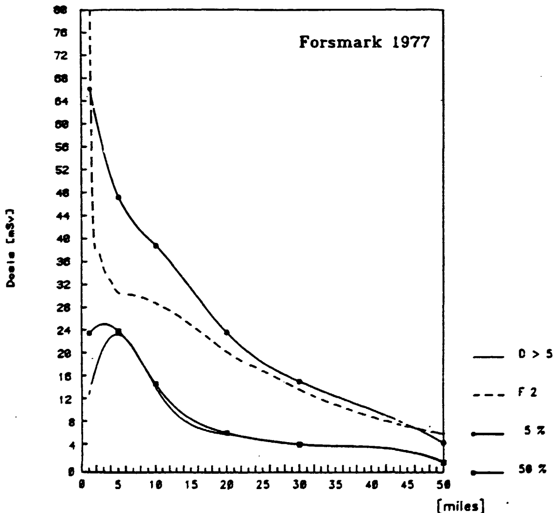
Fig. 2.6. 5 % og 50 % fraktilerne som funktion af afstanden fra værket. Desuden vejr-situationerne Pasquill D med vindhastigheden 5 m/s og Pasquill F med vindhastigheden 2 m/s.
