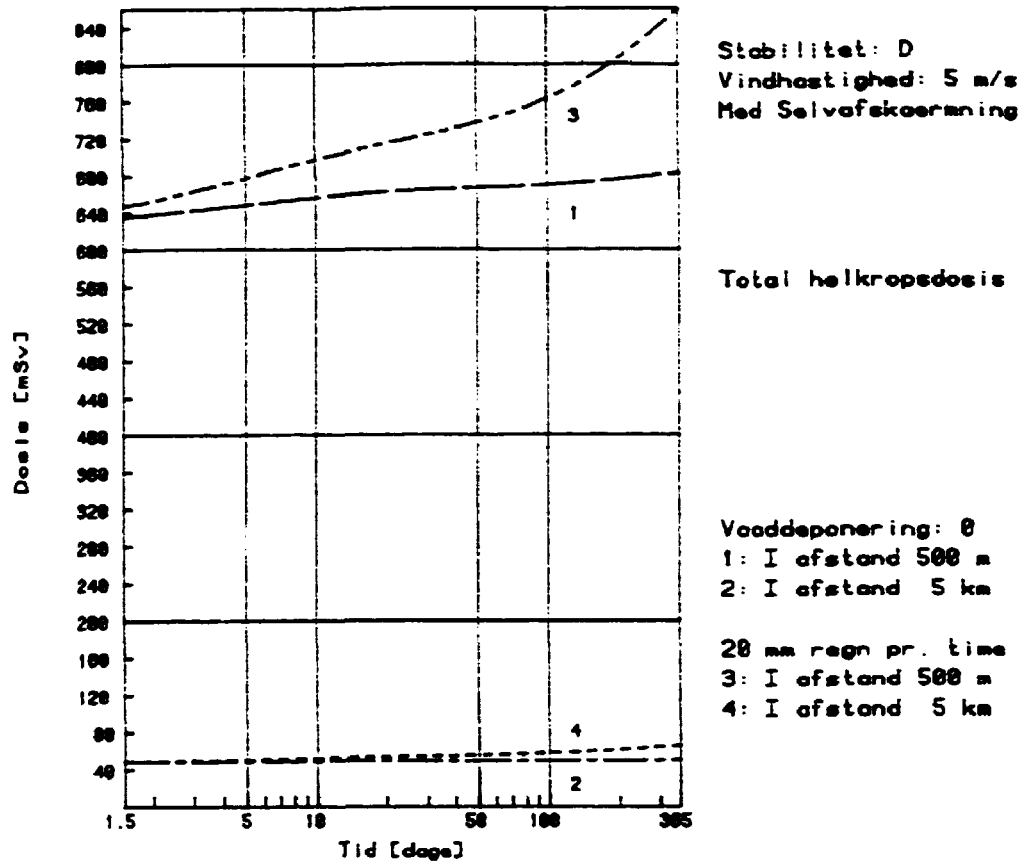
Fig. C.9. Total helkropsdosis ved normal færden i 1 år og indendørs ophold det første 1 1/2 døgn.
