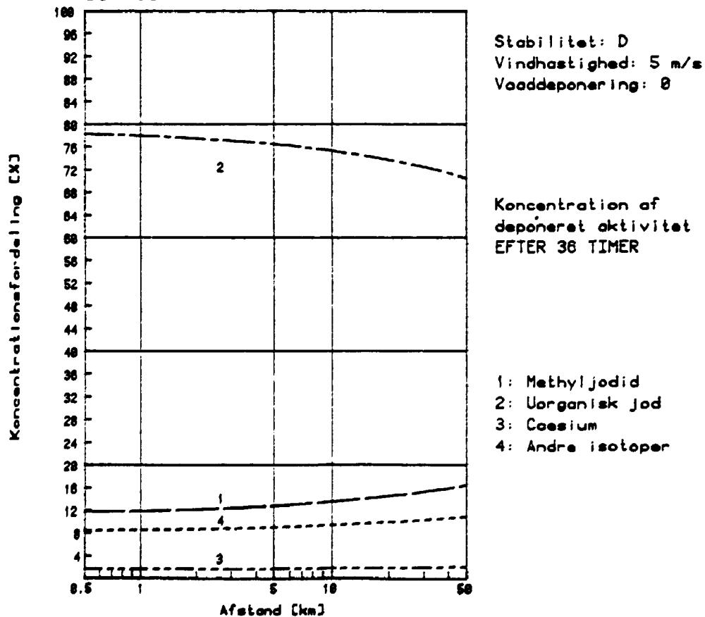
Fig. C.2B. Isotopgrupperfordeling af koncentration af deponeret aktivitet efter 36 timer.
