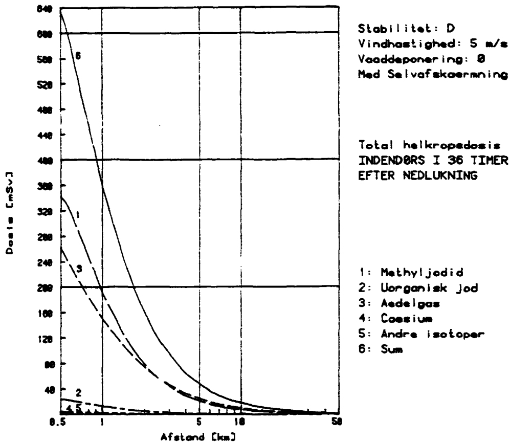
Fig. C.1A. Total helkropsdosis opdelt i isotopgrupper.
