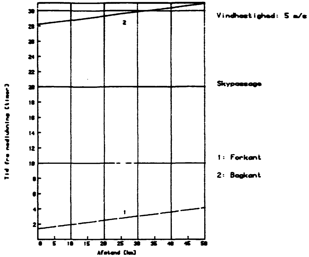
Fig. 4.1. Tidsforløb for skypassage med vindhastighed 5 m/s, som bruges ved stabilitet D.
