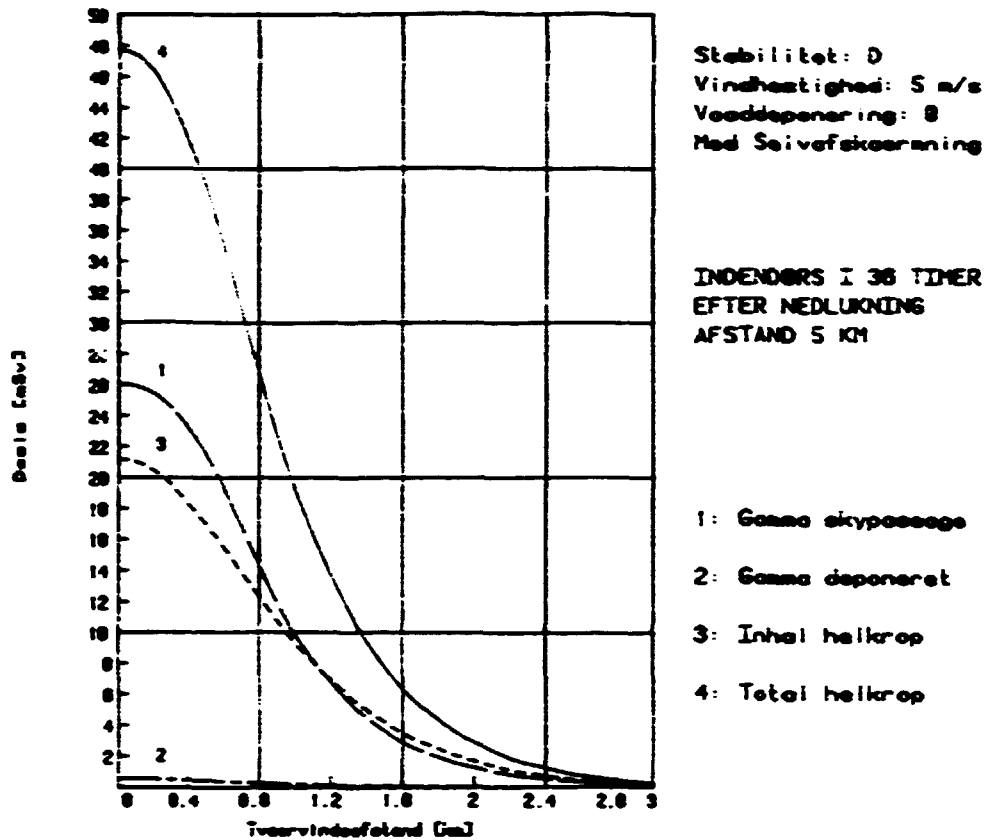
Fig. 5.2. Total helkropsdosis på tværs af centerlinien i afstanden 5 km opdelt i dosiskomponenter.
