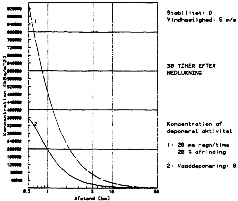
Fig. 5.5. Koncentration af deponeret aktivitet ved 20 mm regn i timen, sammenlignet med kurven uden regn.
