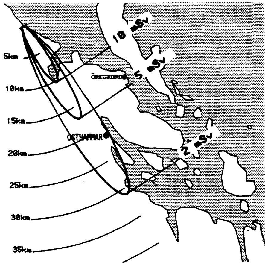
Fig. C.5. Gammadosis tra skypassage ved indendørs ophold.
