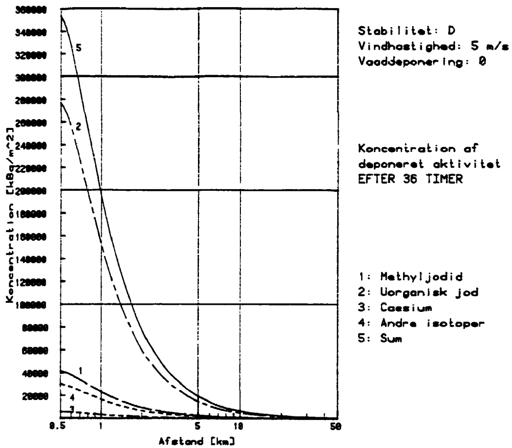
Fig. C.2A. Koncentration af deponeret aktivitet opdelt i isotopgrupper efter 36 timer.
