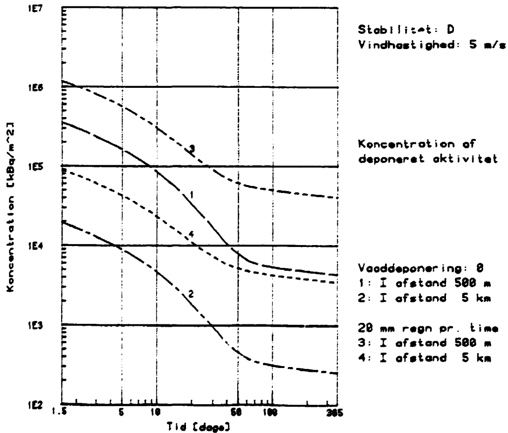
Fig. C.10. Koncentration af deponeret aktivitet i 4 afstande. Efter 36 timer indendørs regnes med normal færden.
