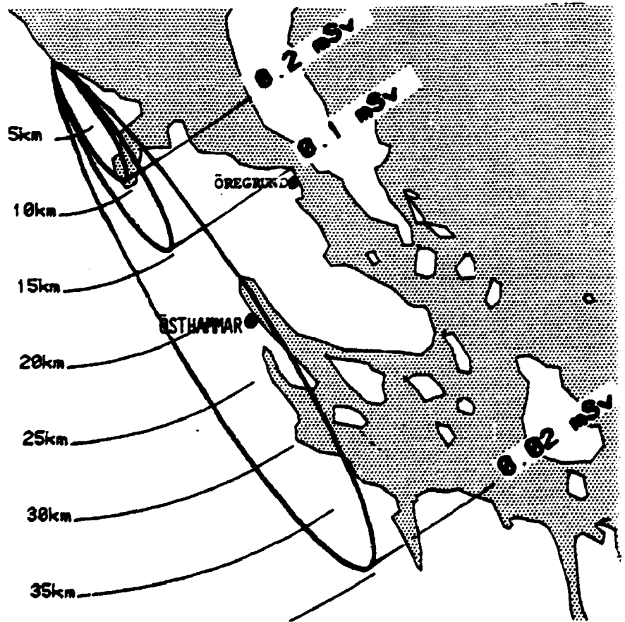
Fig. C.6. Gammadosis tra deponeret aktivitet ved 36 timers indendørs ophold.
