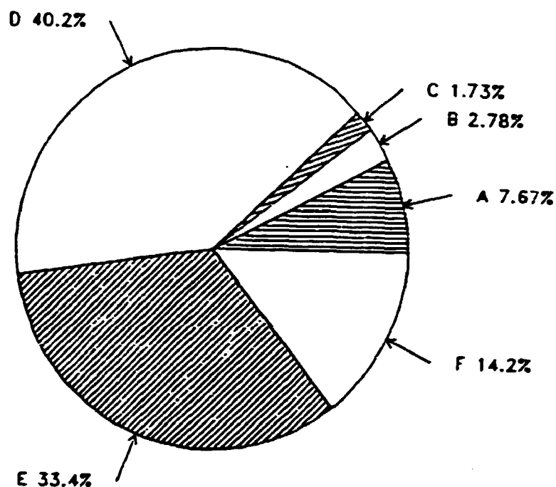
Fig. 2.1. Fordeling af atmosfærisk stabilitet for Forsmark i perioden 23/4-1976 til 26/2-1978. Temperaturgradient fra 2 til 96 m.
