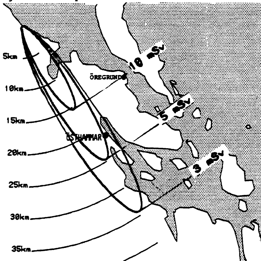
Fig. C.8. Total helkropps-dosis med integrationstid på 50 år.
