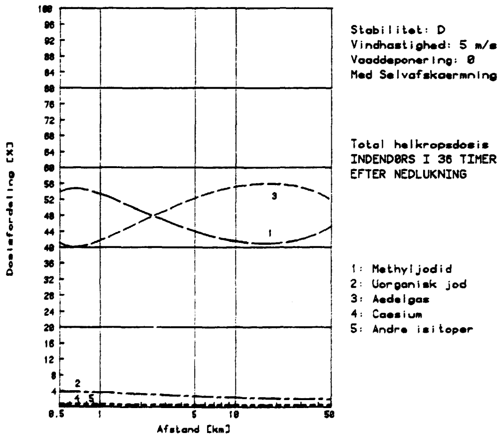
Fig. C.1B. Isotopgruppefordeling af total helkropsdosis.
