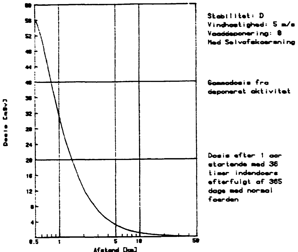
Fig. C.12. Gammadosis fra deponeret aktivitet efter 1 år. Efter 36 timer indendørs regnes med normal færden.
