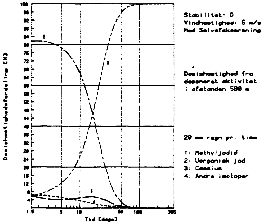
Fig. C.11B. Isotopgruppefordeling af dosisnastighed fra deponeret aktivitet 500 m fra værket.
