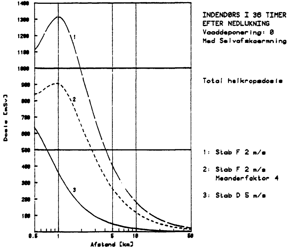
Fig. 5.7. Total helkropsdosis ved stabilitet F og D.
