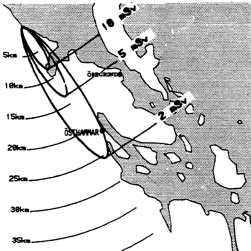
Fig. C.7. Inhalationsdosisbidrag till helkropps-dosis med integrationstid på 50 år.
