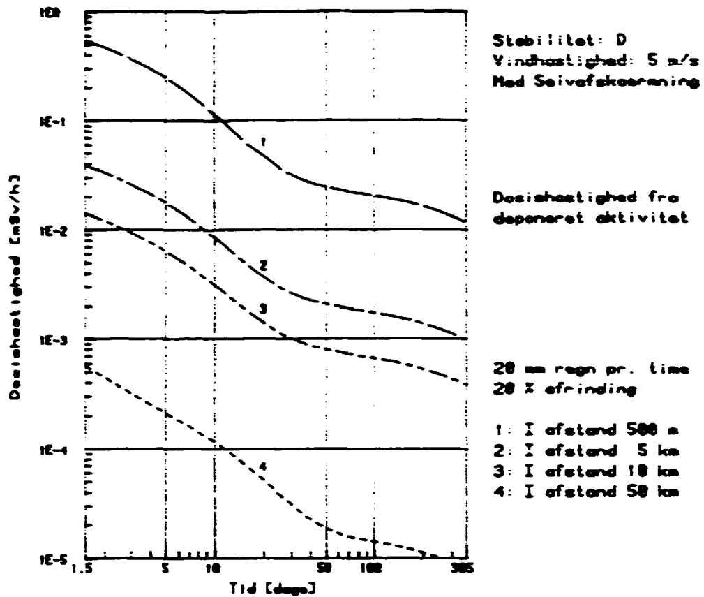
Fig. C.11A. Dosisnastighed fra deponeret aktivitet i 4 afstande ved stabilitet D.
