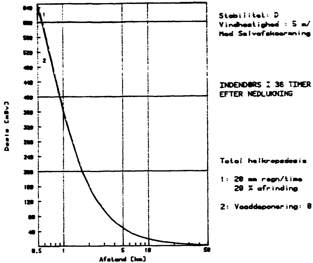
Fig. 5.4. Total helkropsdosis ved 20 mm regn i timen, sammenlignet med kurven uden regn.
