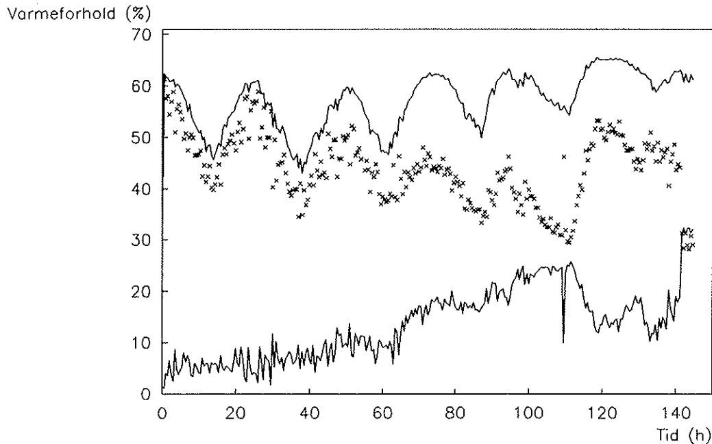
Fig. 4.8. Beregnede (efter fig. 4.7) og målte varmekorhold samt difference som funktion af tiden.
