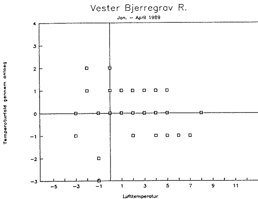
Figur A5.10. Temperaturfaldet gennem anlægget set i relation til måledøgnetts minimale lufttemperatur
