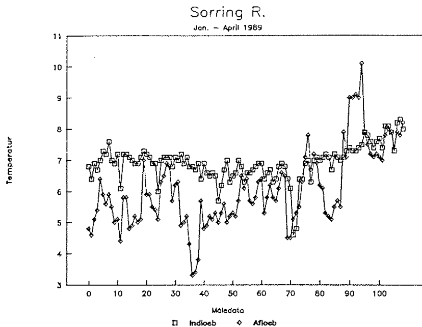
Figur A5.5. De registrerede temperaturer i tilløb og afløb fra renselanlægget
