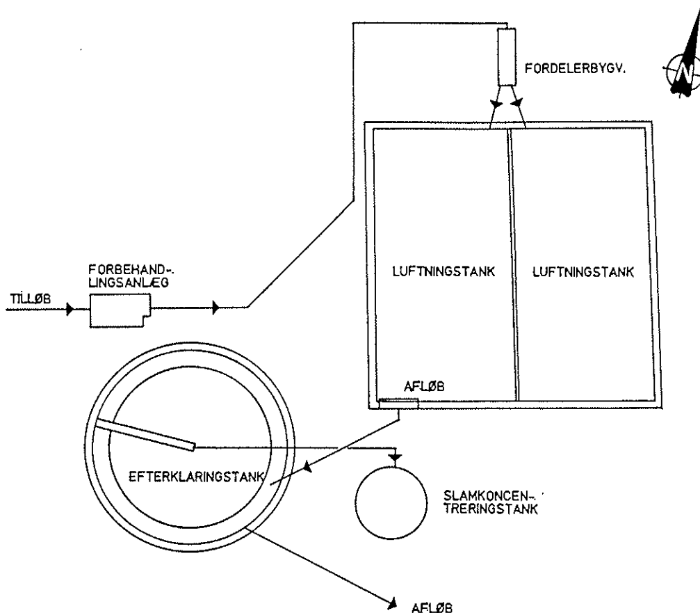
Figur 5.4. Plantegning over Thyborøn-Harboøre renseanlæg
