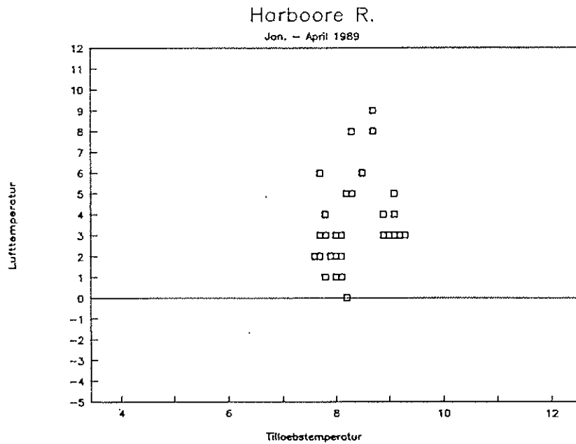
Figur A5.19. Plot af tillobstemperaturen og de minimale lufttemperaturer
