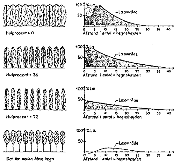
Figur 8.4. Eksempler på hvorledes forskellige hulprocenter indvirker på læhegns intensitet (læprocenten) (ref. 4)
