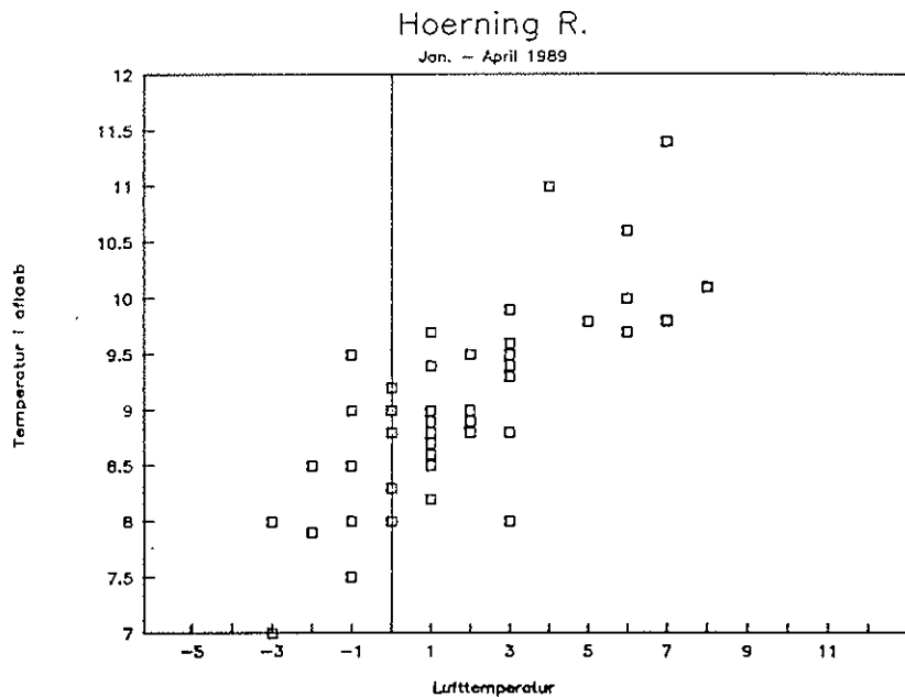
Figur A5.24. Afløbstemperaturen som funktion af lufttemperaturen
