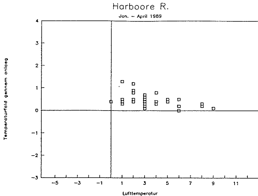
Figur A5.16. Temperaturfaldet gennem anlægget set i relation til måledøgnets minimale lufttemperatur
