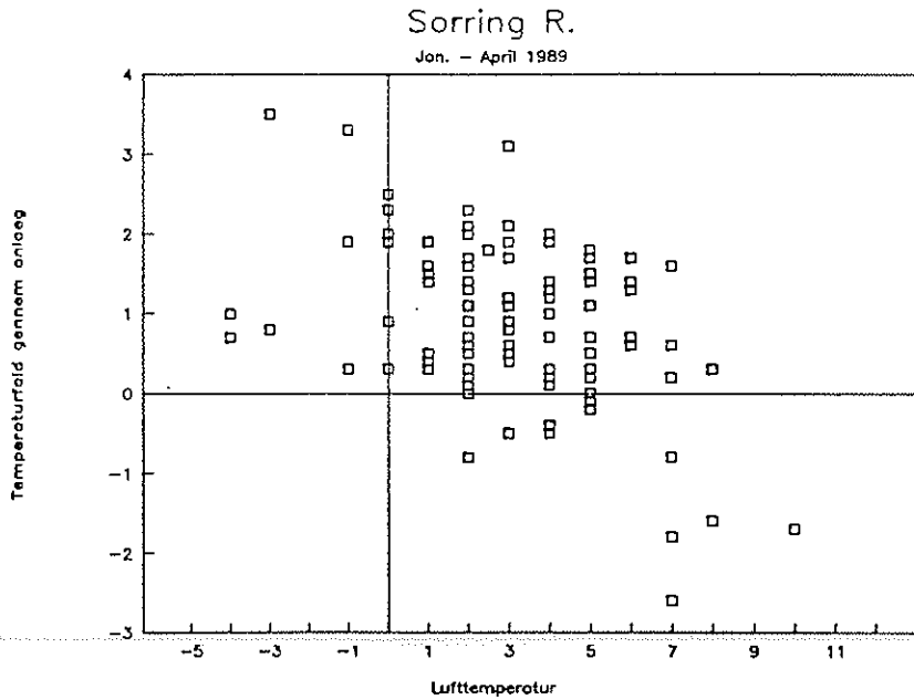
Figur A5.2. Temperaturfaldet gennem anlægget set i relation til måledøgnetts minimale lufttemperatur
