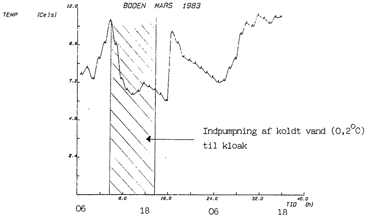
Figur 3.1. Temperatur af tilløbsvand til Bodens avloppsrenningsverk, 9 marts kl. 06 til 10/3 kl. 18 (ref. 15)
