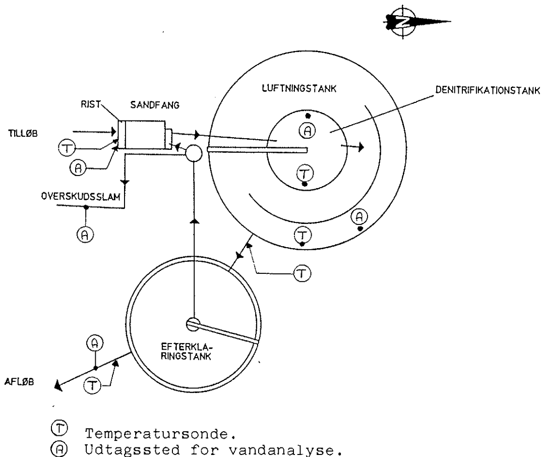
Figur 6.13. Udtagningssteder for vandanalyser på Hørning renselanlæg
