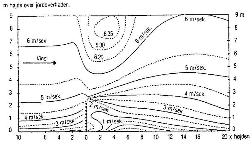
Figur 8.5. Læ i lodret udstrækning. Linier med ens vindhastighed omkring en 2 m høj læskærm med ca. 50% hulareal (ref. 4)
