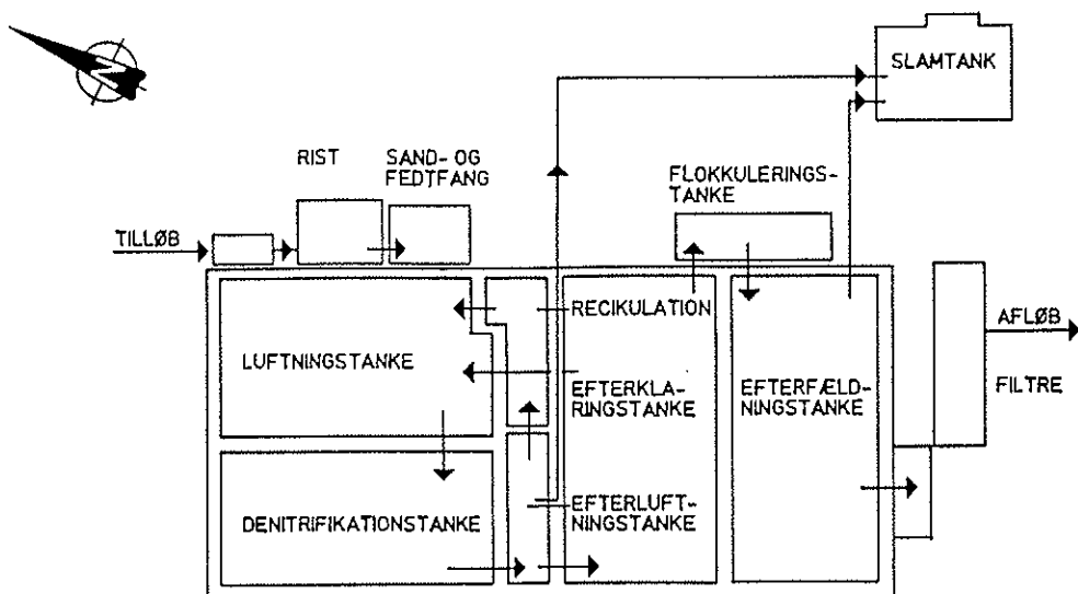
Figur 5.9. Plantegning over Trankær renselanlæg
