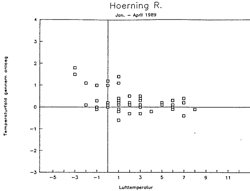
Figur A5.23. Temperaturfaldet gennem anlægget set i relation til måledøgnetts minimale lufttemperatur
