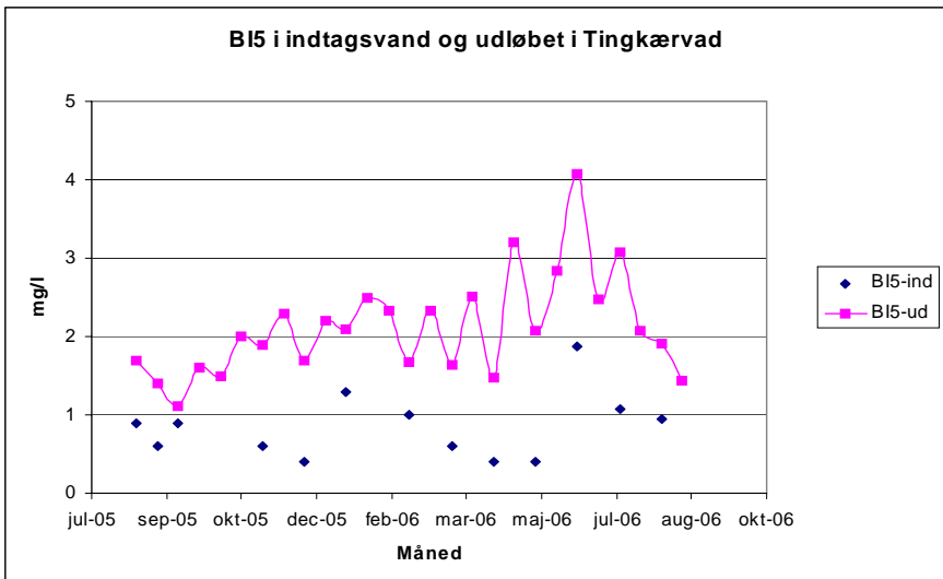
Figur 14 Organisk stof målt som BI 5 koncentrationen (mg/l) i indtagstvandet og i udløbet til Vejle Å i det første måleår på Tingkærøvd Dambrug.
