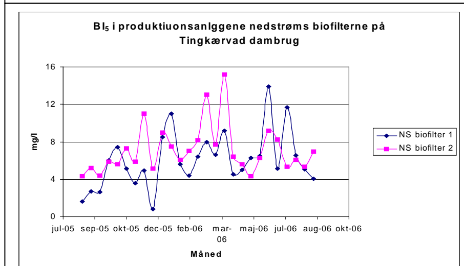
Figur 8 BI_5 koncentrationen (mg/l) i de to produktionsanlæg nedstrøms biofilteret på Tingkæravad Dambrug det første måleår.
