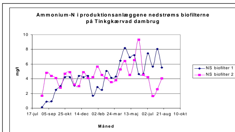
Figur 7 Ammonium-kvælstof koncentrationen (mg/l) i de to produktionsanlæg målt nedstrøms biofilteret på Tingkæravad Dambrug det første måleår.
