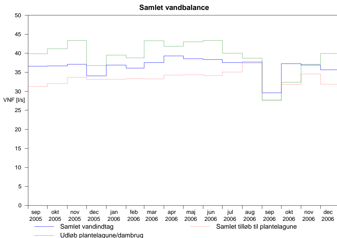
Figur 5 Samlet vandbalance over Tingkæravad Dambrug, månedsmiddel (l/s)
