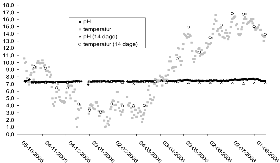
Figur 4 Gennemsnit pr. døgn for temperatur og pH inden beluftning i udløbet fra Tingkæravad Dambrug. Endvidere er der angivet målinger foretaget hver 14. dag (øjebliksværdier med håndholdte instrumenter) på samme sted.
