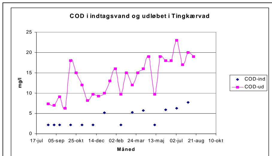
Figur 15 Organisk stof målt som COD koncentrationen (mg/l) i indtagstvåndet og i udløbet til Vejle Å i det første måleår på Tingkæravad Dambrug.
