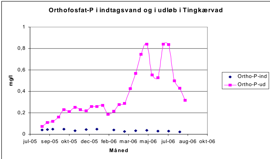
Figur 12 Orthofosfat-fosfor koncentrationen (mg/l) i indtagstvandet og i udløbet til Vejle Å i det første måleår på Tingkærøvd Dambrug.
