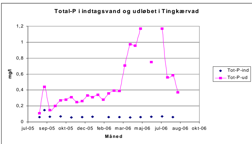
Figur 13 Total-fosfor koncentrationen (mg/l) i indtagstvandet og i udløbet til Vejle Å i det første måleår på Tingkærøvd dambrug
