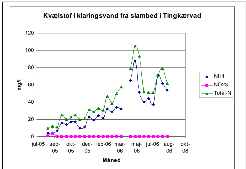
Figur 17 Koncentrationen af ammonium-N, nitrit/nitrat-N og total-N i klaringsvandet fra slambassinet, der løber til plantelagunen på Tingkærvad Dambrug i det første måleår.
