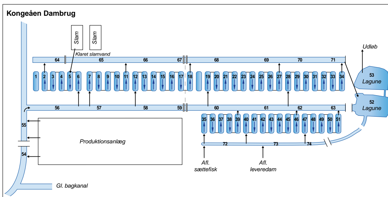
Figur 16.2.2.1 Principskitse af plantelagunen på Kongeåens Dambrug. Se teksten for forklaring af symboler.
