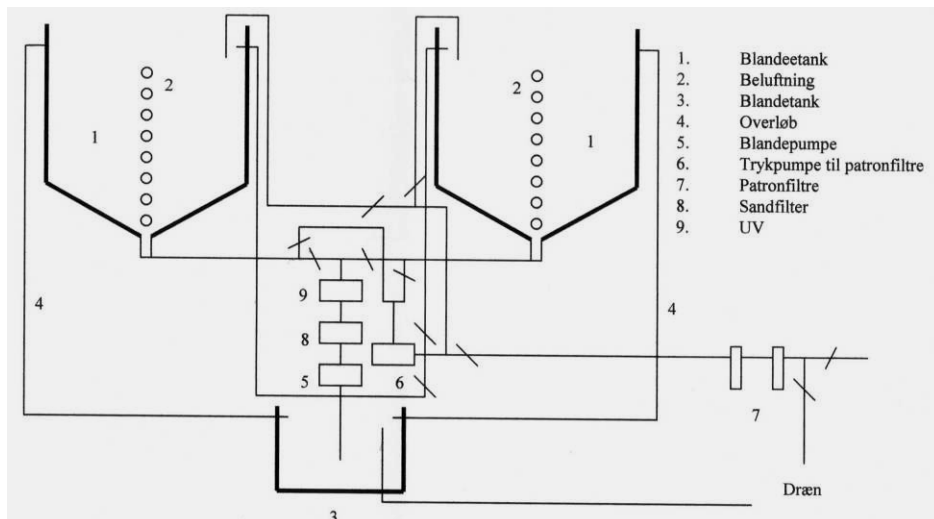
Figur 3.3. Anlæg til produktion af kunstigt saltvand. (Foto: C. Graver, tegning: Billedlund Aquakulturservice)
