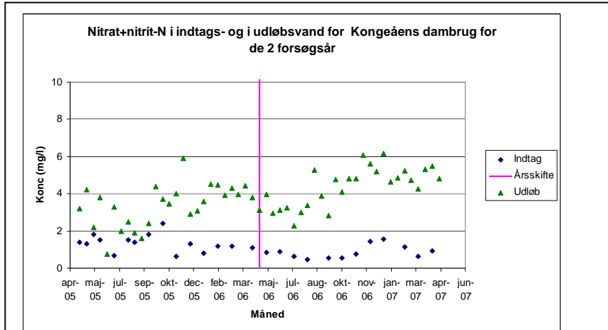
Figur 26 Nitrat+nitrit-kvælstof koncentrationen (mg/l) i indtagsvandet til Kongeåens Dambrug og i afløbet fra dambruget til Kongeåen i første og andet måleår.
