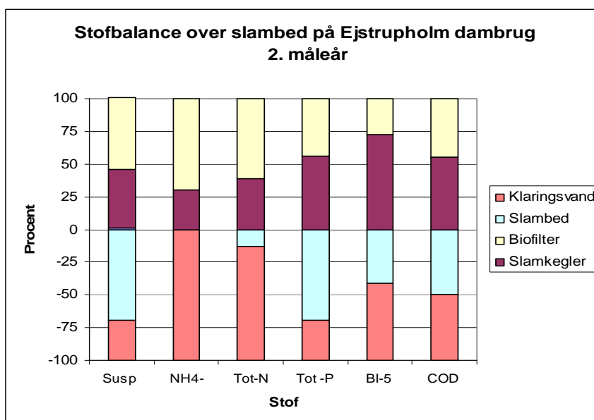
Figur 30 Stoffjernelse over slambassiner på Ejstrupholm Dambrug det andet måleår. Bidragene kommer fra biofiltre og slamkegler i produktionsanlægget. Stoffindholdet i klaringsvandet angiver stoftabet fra slambassinerne.
