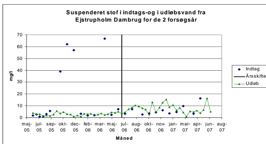
Figur 29 Suspenderet stof-koncentrationen (mg/l) i indtagsvandet til Ejstrupholm Dambrug og i afløbet til Holtum Å i første og andet måleår.
