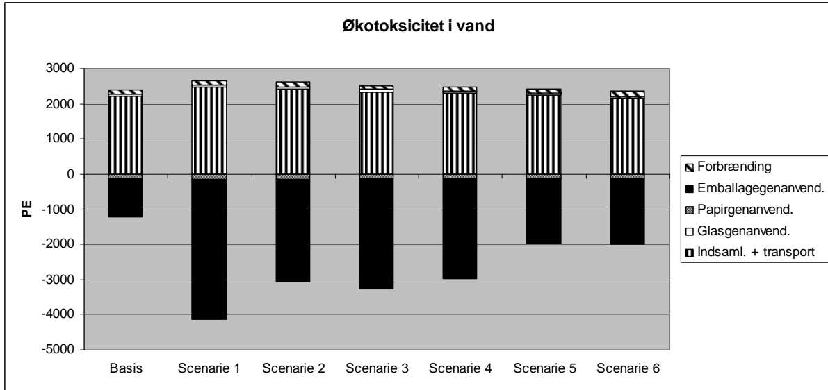
Figur 7. Potentiel økotoxicitet i vand i basisscenariet og scenarie 1-6 fordelt på behandlingsfaser.
