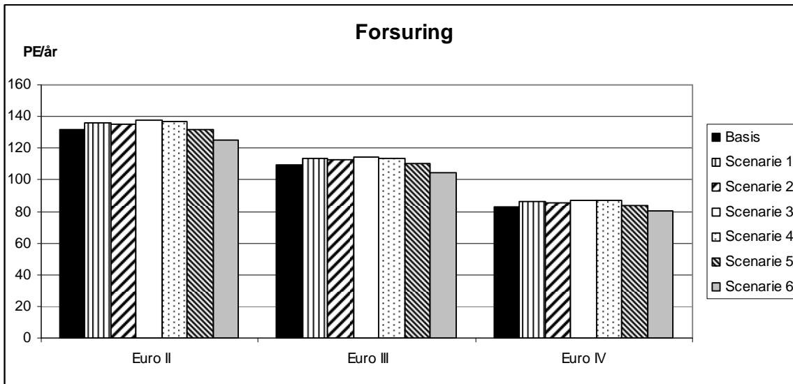
Figur 30. Potentiel forsuring ved indsamling for Euro-standarder II, III og IV.
