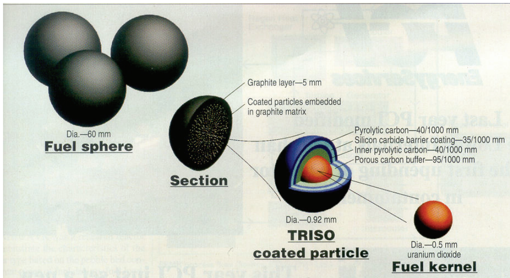
Figur 2.2. PBMR brændselsdesign.
