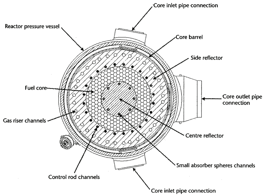
Figur 2.4. Vandret snit af PBMR-design.
