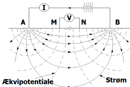
Figur 1. Strømbaner og ækvipotentialer overflader for en homogen isotropisk jord. A og B er strømelektroder og M og N potentialelektroder.
