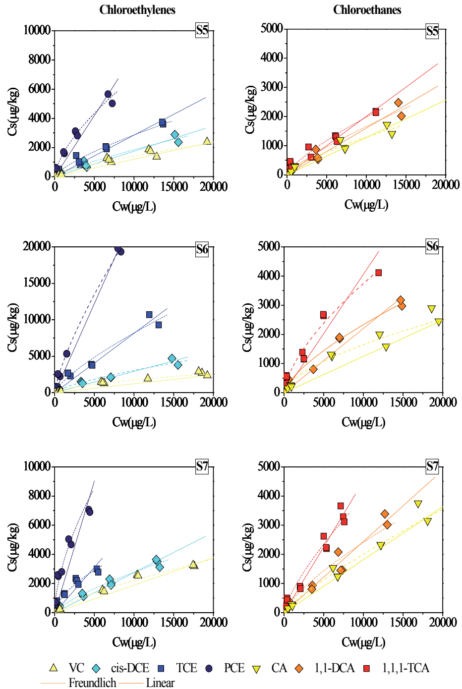
Figur 1: Sorptionsisothermer for sorption af chlorerede ethener og ethaner til 3 morænelersprøver fra lokaliteten Vadsbyvej. S5 fra oxideret zone og S6 og S7 fra reduceret zone.
