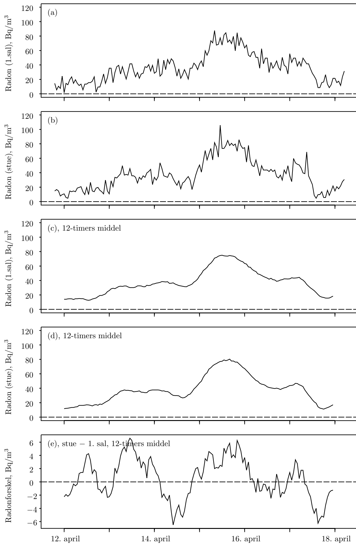
Figur A.24. Kontinerte radonmålinger i stue og på første sal.
