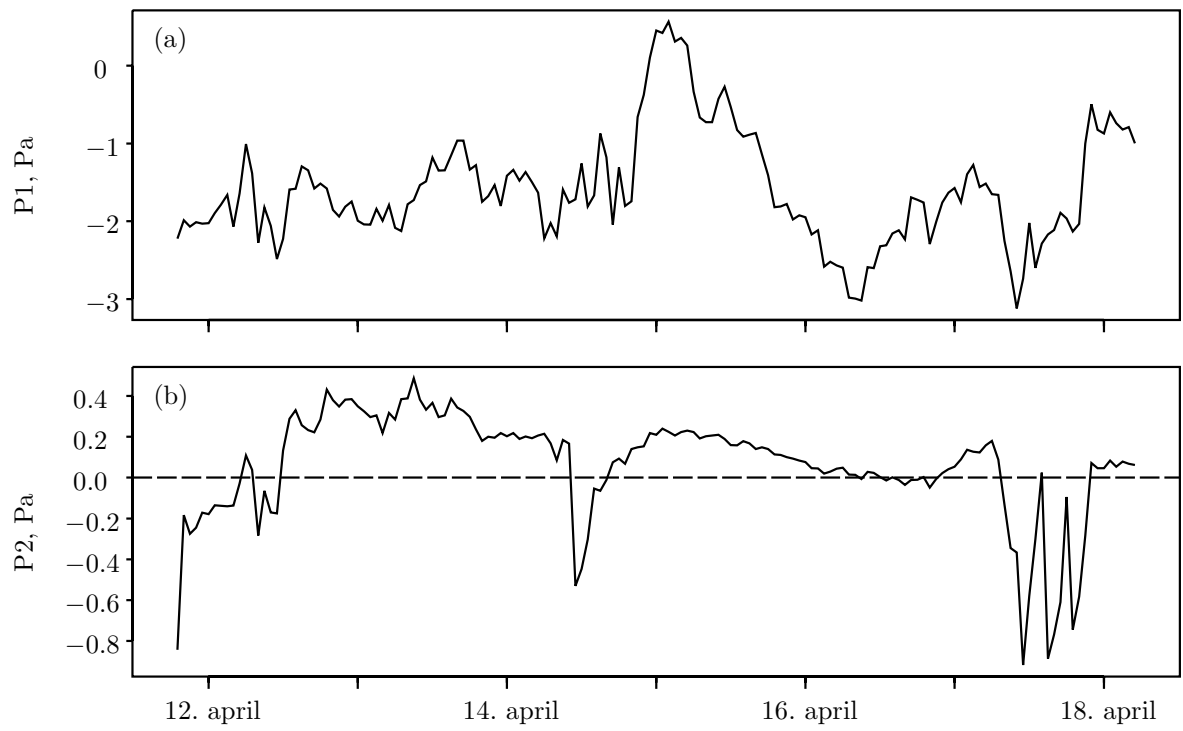
Figur A.25. Kontinerte målinger af differenstrykkene P1 (mellem probe TB03 og hus) samt P2 (mellem det kapillarbrydende lag og hus).
