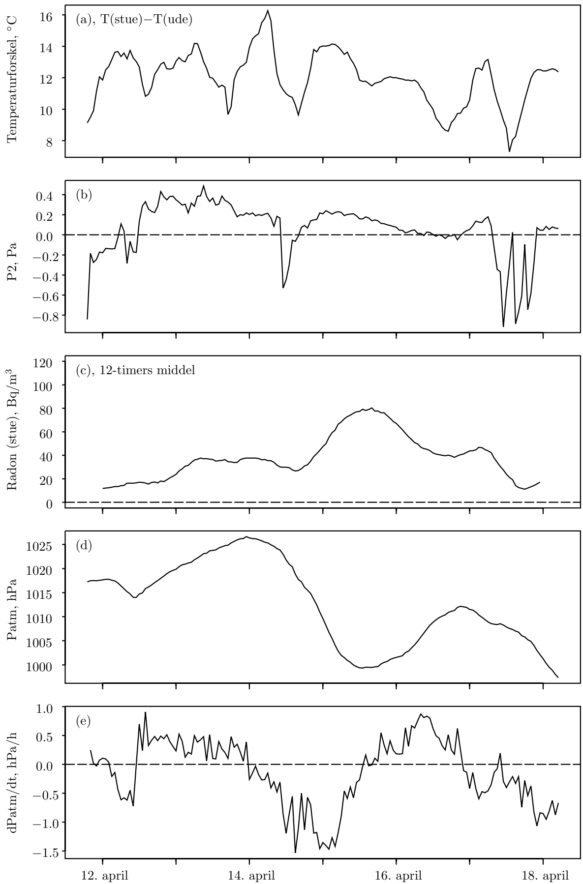
Figur A.23. Oversigt: (a) Temperaturdiff., (b) trykdiff. mellem Gulv1 og hus, (c) radon i stuen, (d) atm. tryk, og (e) ændringshastighed af atm. tryk.
