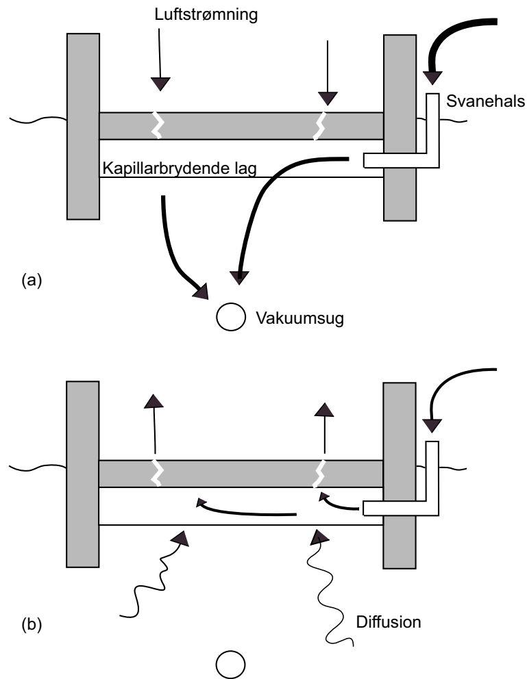
Figur 10. Sempel skematisk model for luftstrømning og radontransport omkring huset med vakuumanlægget tændt (a) og slukket (b). Det formodes, at svanehalsen spiller en vigtig rolle for lufttilførslen til det kapillarbrydende lag.
