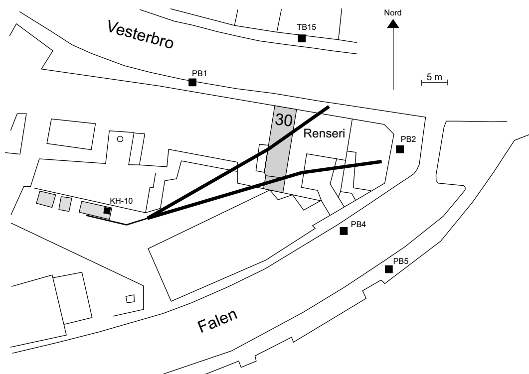
Figur 2. Skitse af området omkring den undersøgte ejendom (gråtonet). De sortmalede firkanter (PB1, PB2 etc.) viser, hvor der er foretaget poreluftmålinger af radon. De horisontale rør til vakuumelektraktion danner et "v". Punktet KH-10 angiver stedet for radonmåling af den opsugede luft før filtret med aktivt kul.
