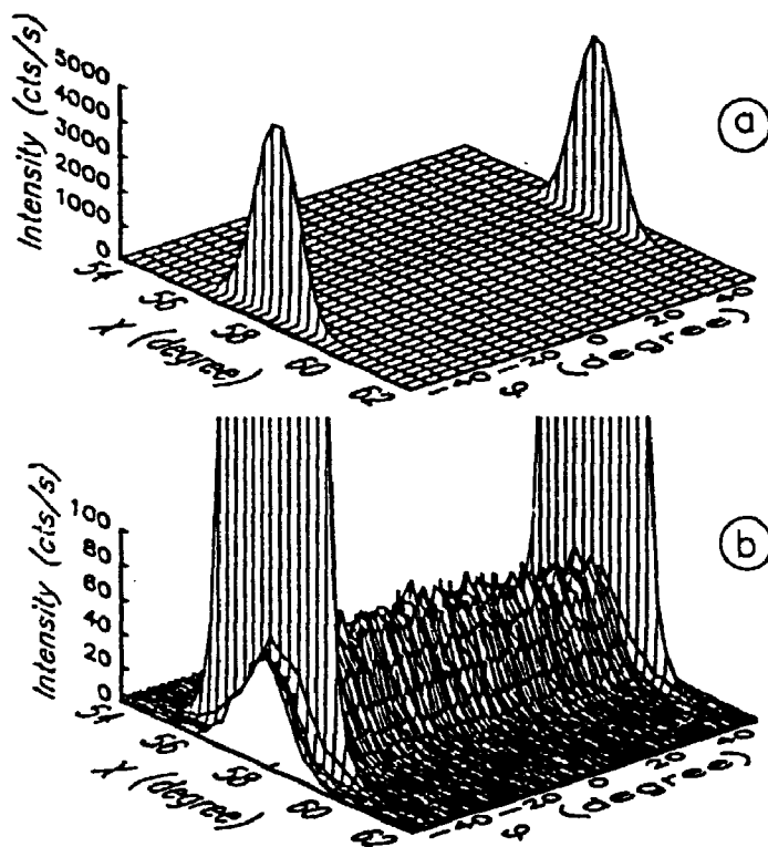
Figur 9: (a) Euler fire-cirkel røntgendiffractions undersøgelser af \text{Bi}_2\text{Sr}_2\text{CaCu}_2\text{O}_{x+n} (115) Bragg refleksen fra en tyndfilm fremstillet på \text{NdGaO}_3 (001) som funktion af Euler vinklerne \chi og \varphi (for flere detaljer om Euler fire-cirkel geometrien, se EFP90-rapporten: Andersen, N.H.(1992)). For fuldt epitaksielle film forventes to skarpe toppe ved \chi = 57.5^\circ , og \varphi = -45^\circ og \varphi = 45^\circ , som observeret. (b) En nøjere analyse viser imidlertid, at der mellem disse dominerende toppe også er en homogen fordeling af (115) spredningsintensitet for alle \varphi -værdier, svarende til at en del af filmen er tilfældigt orienteret i filmplanen.
