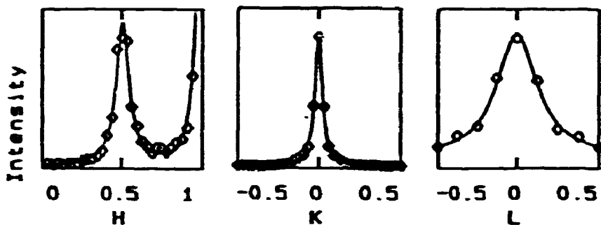
Figur 4: Diffractionsprofiler af (1/00) superstruktur refleksen langs de tre krystallografiske akser, beregnet ved Monte Carlo simuleringer baseret på en tre-dimensionel version af den såkaldte ASYNNI model. De beregnede korrelationslængder svarer til middel-dimenss størrelser med udstrækningen 10a , 20b og 3c .
