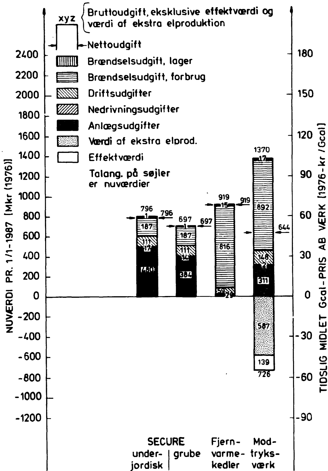
Fig. 7: Udgifter til SECURE samt udgifter til oliefyrede fjernvarmekedler og til et kulfyret modtryksværk. Varmeeffekt 200 \text{ MW}_t . Faste brændselspriser. Udgifter til transmissionsledninger er ikke medtaget.
