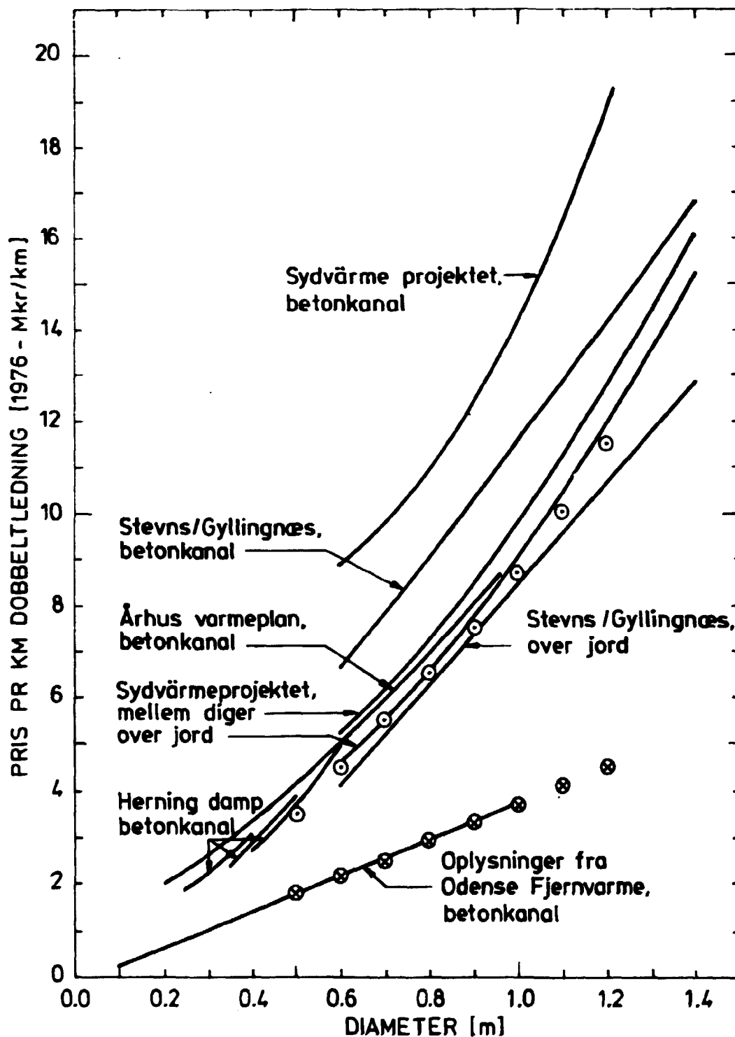
Fig. 3.4: Kontraktpriser for rørledninger
