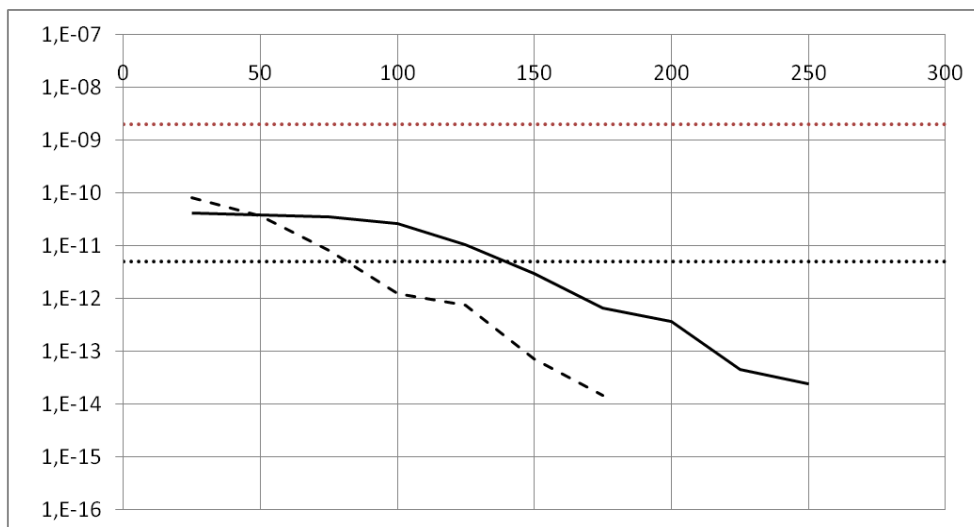
Figur 2. Sandsynlighed pr kørt km for at en person i et køretøj mister livet pga. isafkast fra en vindmølle som funktion af afstanden til en vej. Fuldt optrukken kurve: vindmølle i drift - stiplet kurve: vindmølle stoppet.
