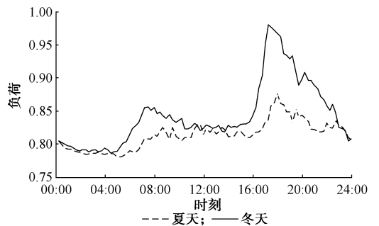
图 5 某配电系统负荷曲线
