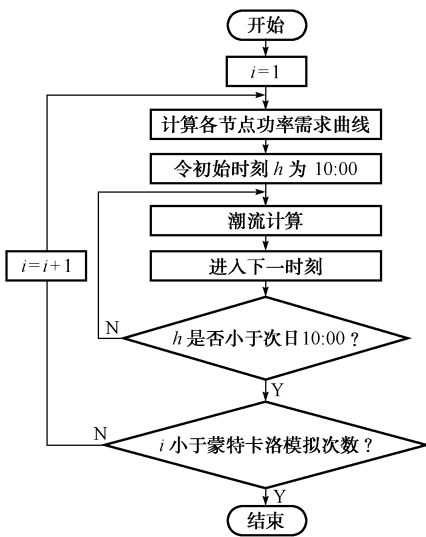
图 3 配电系统的蒙特卡洛仿真分析
