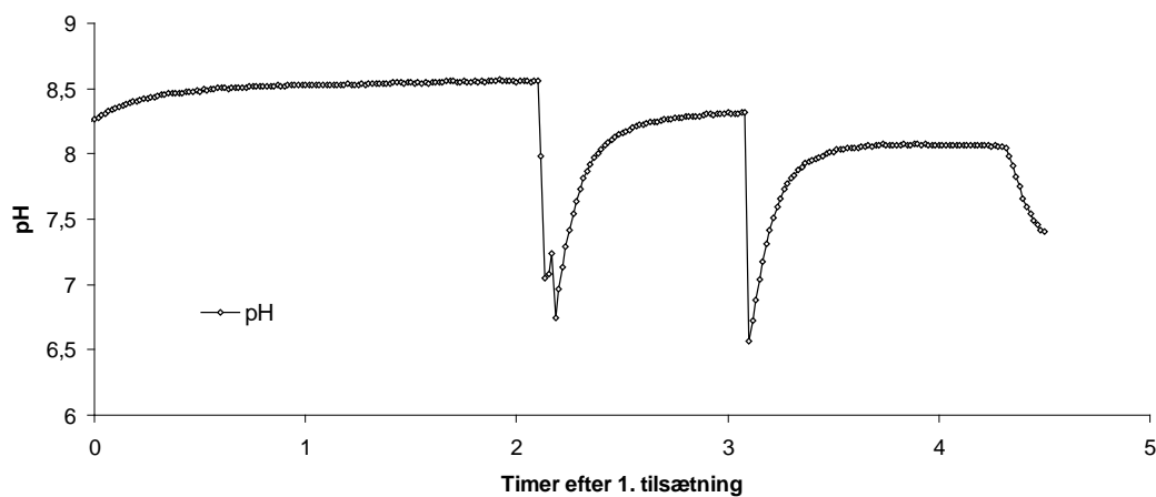
Figur 5.7. Logningsdata ved forsøg med gentagne nitrit tilsætninger og sænkelse af alkalinitet. Tilførsel til reaktoren afbrydes ca. \frac{1}{2} før første tilsætning ( t=0 ); efter ca. 2 og 3 timer tilsættes saltsyre for at reducere alkaliniteten. Efter knap 4\frac{1}{2} time åbnes der atter for vandtilførsel med ammoniumklorid.
