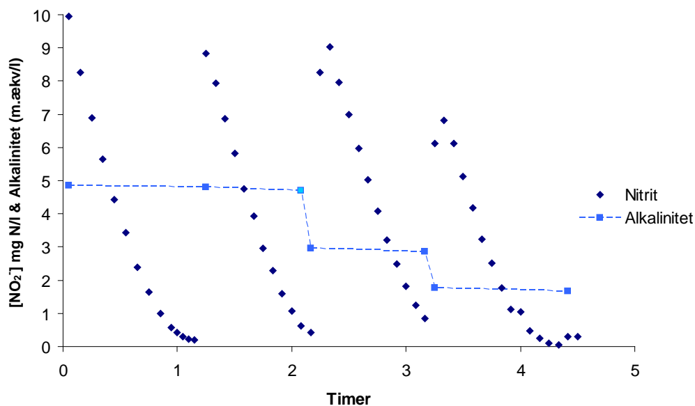
Figur 5.6. Resultater af gentagne \text{NaNO}_2 tilsætninger til en lukket reaktor med BiofilmChip filter-elementer ved forskellige målte alkalinitetsbetingelser. Vandtemperatur 19,5 C, COD ~ 20 mg/l; pH og iltdata logget og afbildet særskilt. NB: Alkalinitet er bestemt ved titrering (undtagen vandprøve efter 2. tilsætning (lyseblå), og målt med sticks.
