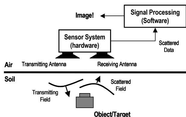
Figur 1 Jordradaren og tilhørende signalbehandlingssystem.
