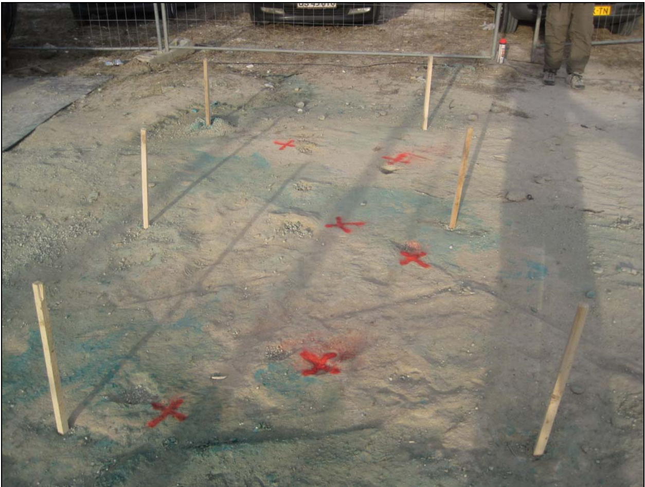
Figur 2 Foto illustration af placering af injektionspunkter (pæle) og planlagte ROST sonderinger (krydser) i injektionsfeltet
