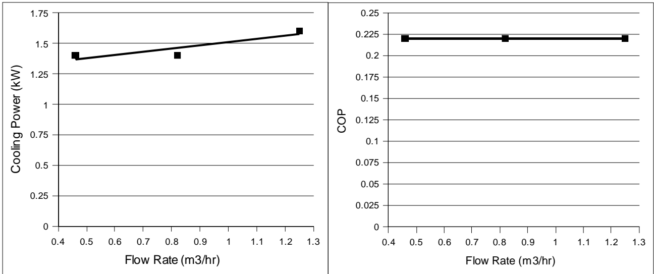
Figure 8: Effect of coolant flow rate on the system performance Figure 8: Influence du débit d'eau de refroidissement sur les performances du système
