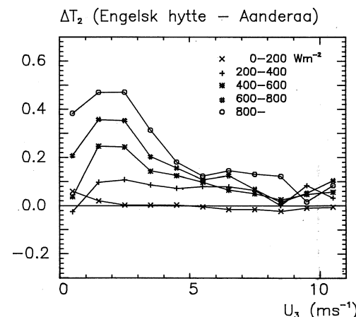
Fig. 3. Middeltemperaturforskellen mellem engelsk hytte og Aanderaa skærm som funktion af den kortbølgede indstråling og vindhastigheden i 3 m. Jylex, juni 1983 - august 1984.
