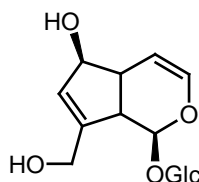
6; Aucubin
