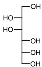
1; Mannitol
