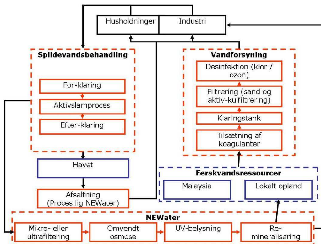
Vandkredsløbet i Singapore. Skitseret efter oplysninger fra (PUB 2006)
